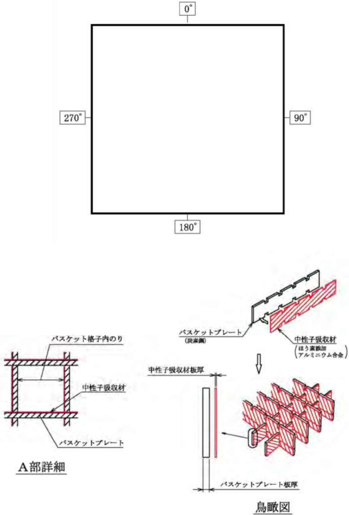
第1図 バスケット構造図
