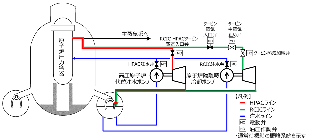
第 57-7-9 図 RCIC 及び HPAC 概略システム図
