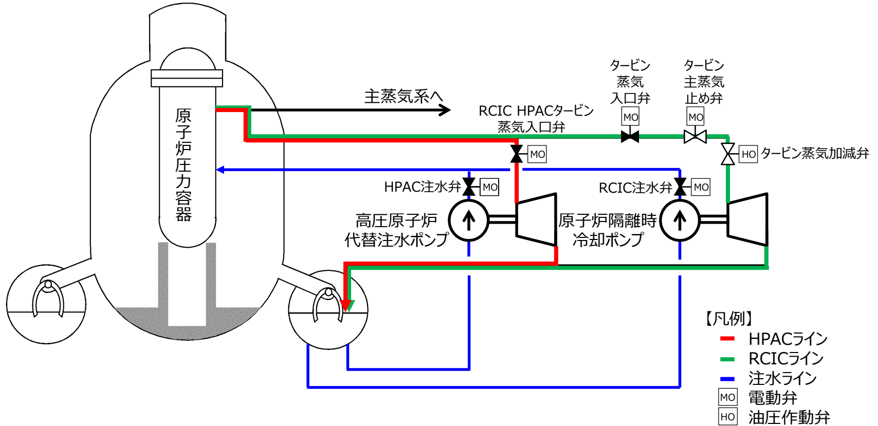
図1 RCIC及びHPAC 概略系統図
