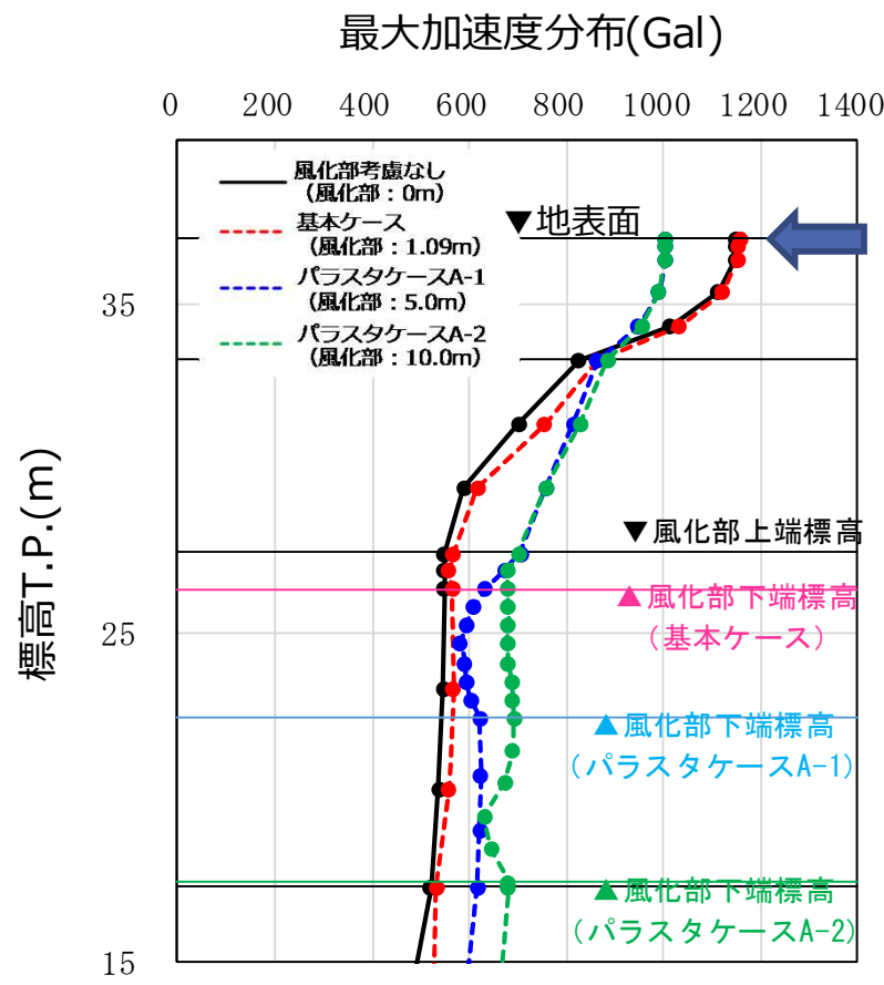
図 最大加速度の深度分布
