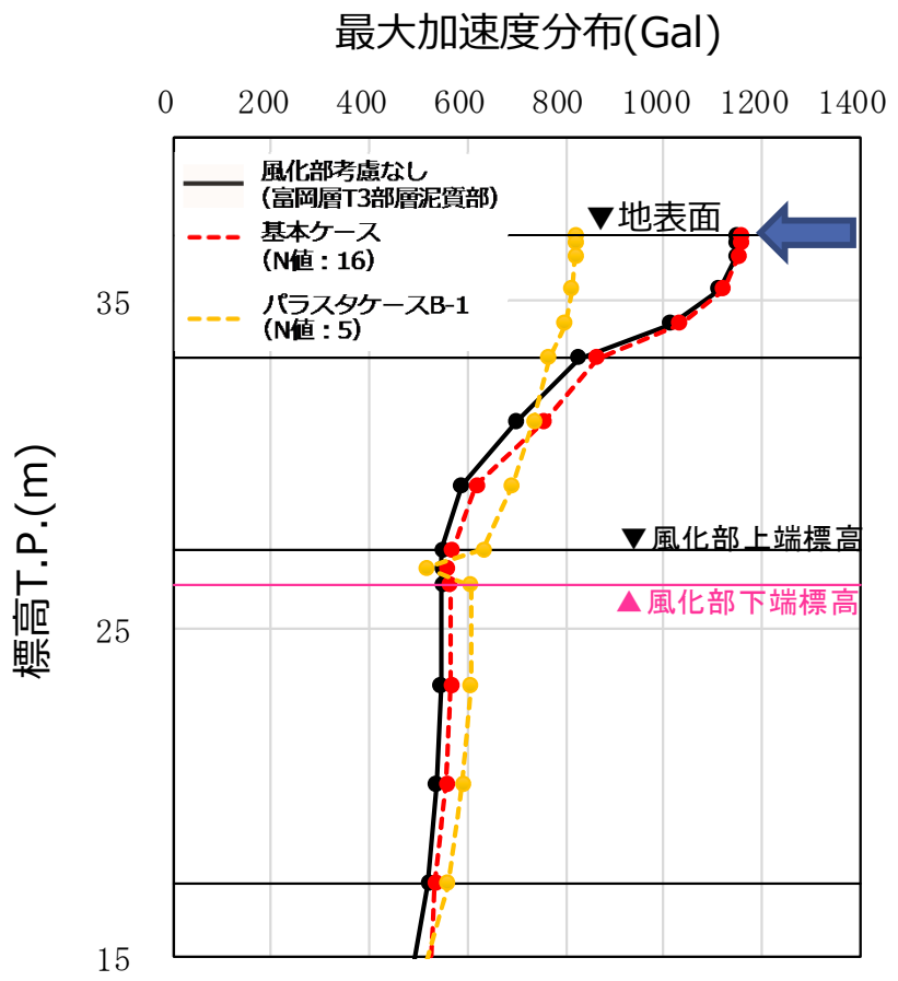
図 最大加速度の深度分布
