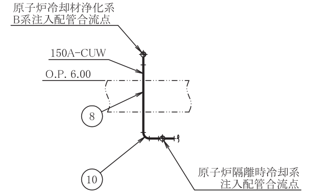
B~B矢視図
