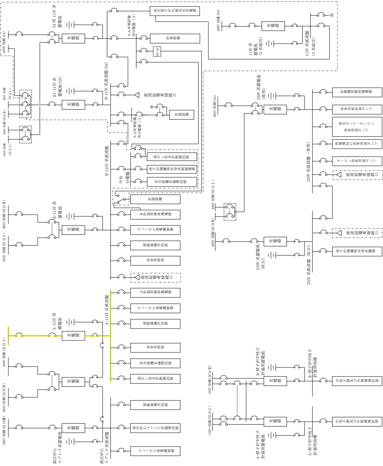
第 1.14-40 図 非常用直流電源喪失時の A-115V 系直流受電 概要図
