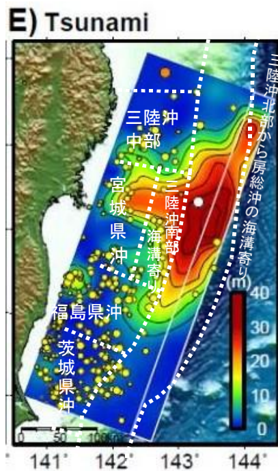
津波インバージョン解析 (Koketsu et al. (2011)に加筆)
