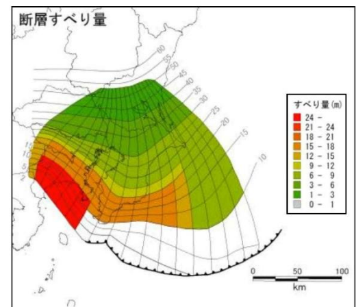
相模トラフ沿いの最大クラスの地震(ケース1(Mw 8.7))
