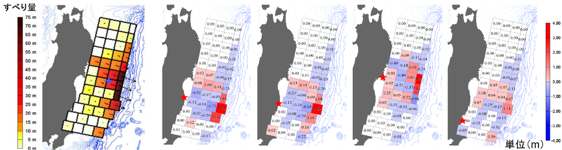
原子力サイトの沖合150m水深点の最大波高における小断層の波高内訳 (杉野他(2013))
