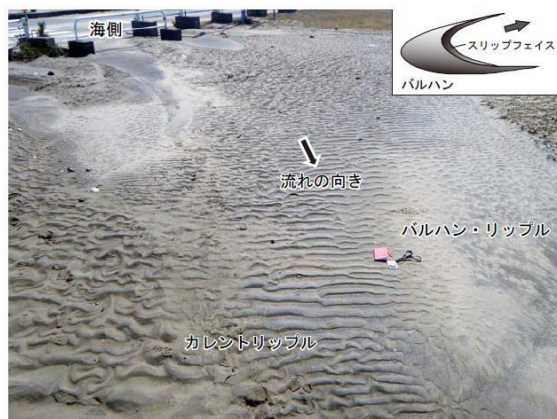
図5 図. 道路の分離帯に形成されたリップルを持つ津波堆積物 (2011/3/13)。海岸から400 m 付近の遡上流による堆積物。淘汰の良い細粒砂層からなり、層厚は最大で約10 cm。リップルの波長は長いもので10 cm。写真中央には直線状のカレントリップル、左手には舌状のカレントリップル、右手には三日月形のバルハンが見られる。活断層・地震センターのHPより転載。
