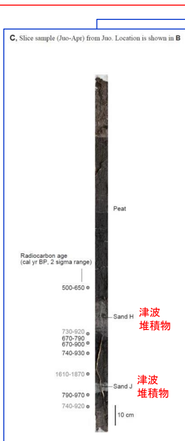
コアの構造とC14年代
