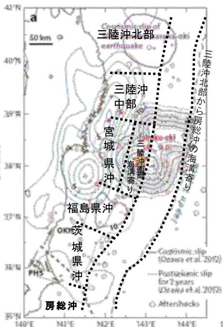
陸上・海上のGPS及び水圧計データに基づく2011年東北地方太平洋沖地震のすべり量分布(黒線) (Ozawa et al. (2012)に加筆)
