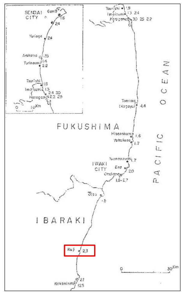
1960年チリ地震津波による福島県～茨城県の津波の高さ分布図 (チリ津波合同調査班(1961)に加筆)
