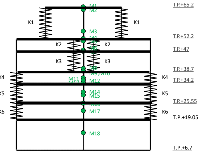
有限要素モデル
