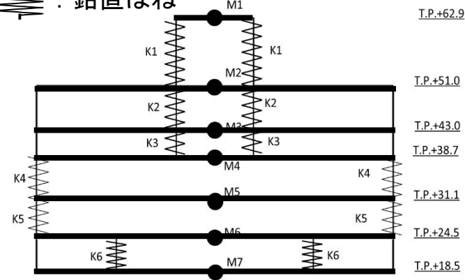
有限要素モデル
