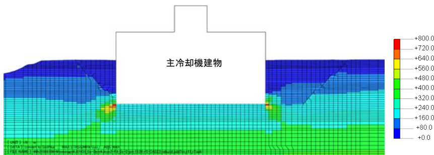
最大せん断応力(kN/m 2 )
