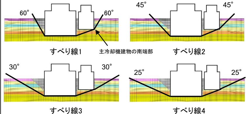
解析モデル(A-A'断面)
