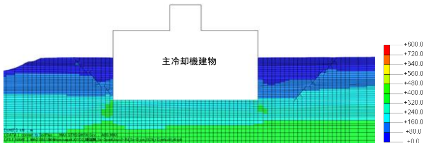
最大せん断応力(kN/m 2 )
