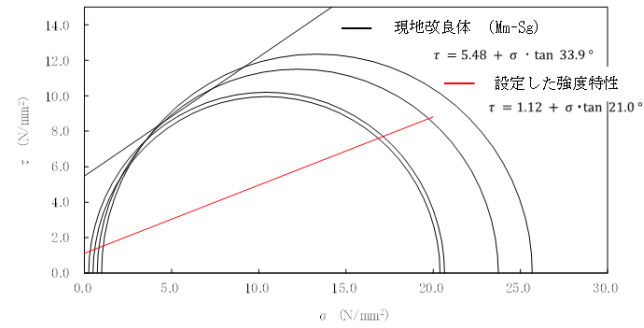
現地改良体 Mm-Sg (砂礫層)
