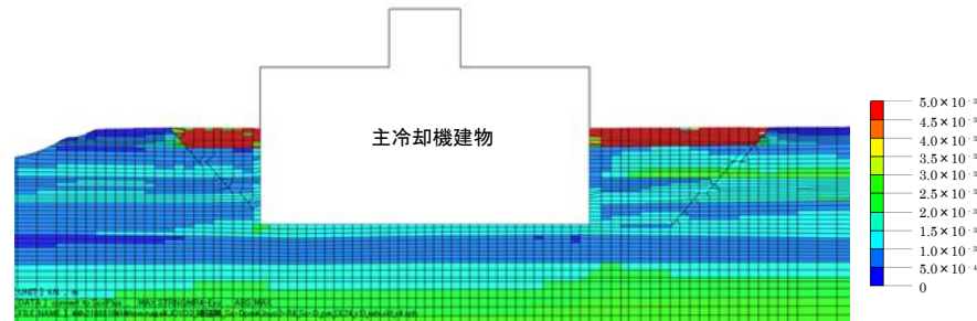
最大せん断ひずみ(-)
