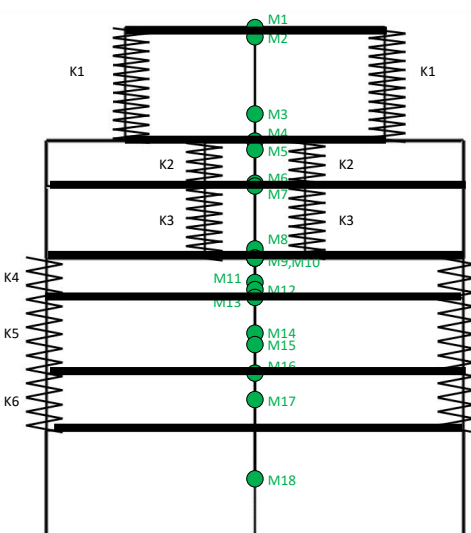
基礎底面 有限要素モデル (水平・鉛直同時加振モデル)
