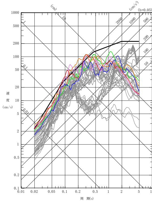
EW成分
