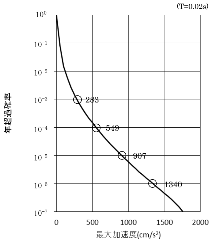
水平成分
