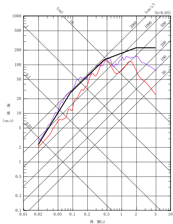
水平成分
