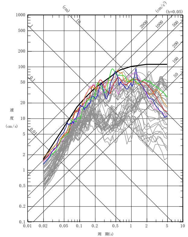
UD成分
