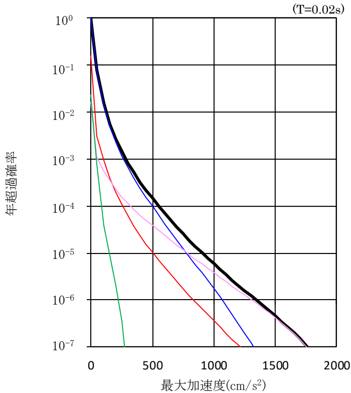
水平成分
