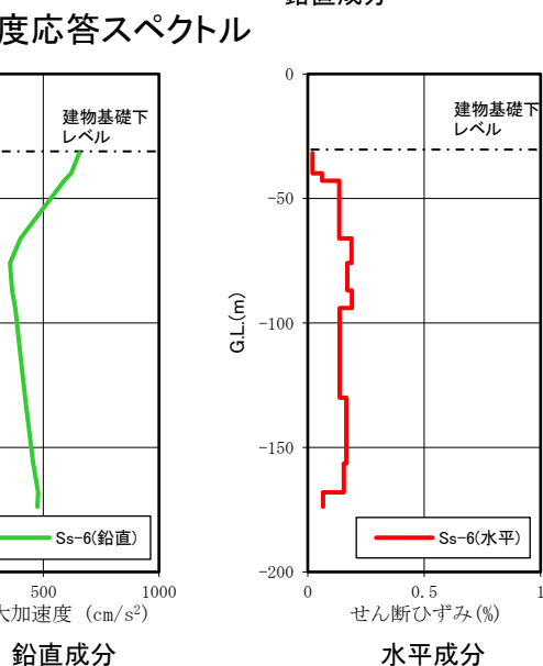
せん断ひずみ分布
