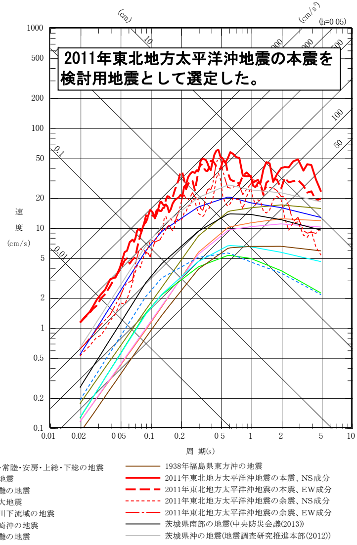
プレート間地震の地震動の応答スペクトル【水平】 (Noda et al.(2002)の手法に補正係数を考慮)
