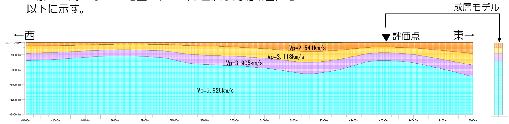
2次元FEMモデル（東西断面）
