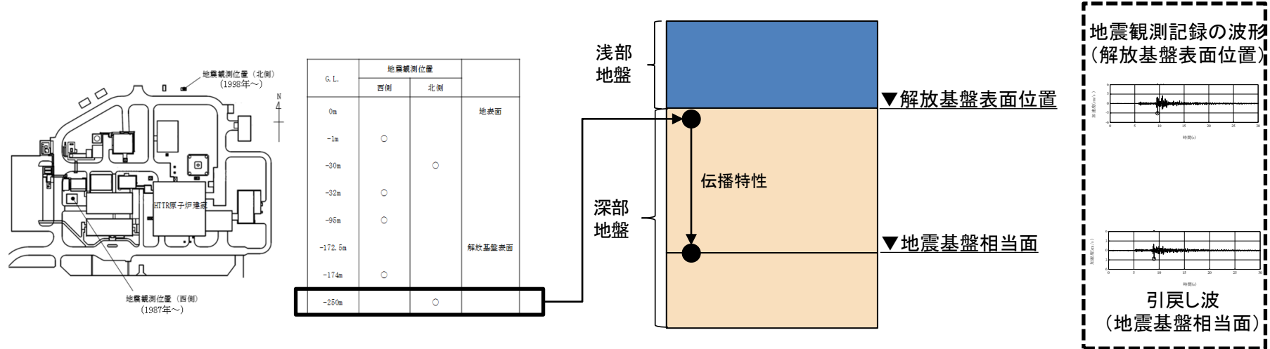
大洗研HTTR 地震観測位置
