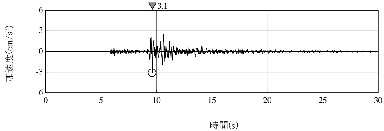
水平成分
