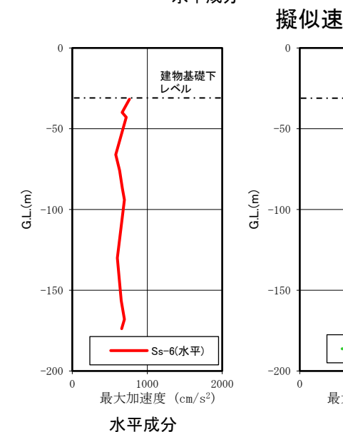
最大加速度分布
