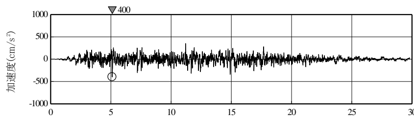
鉛直成分
