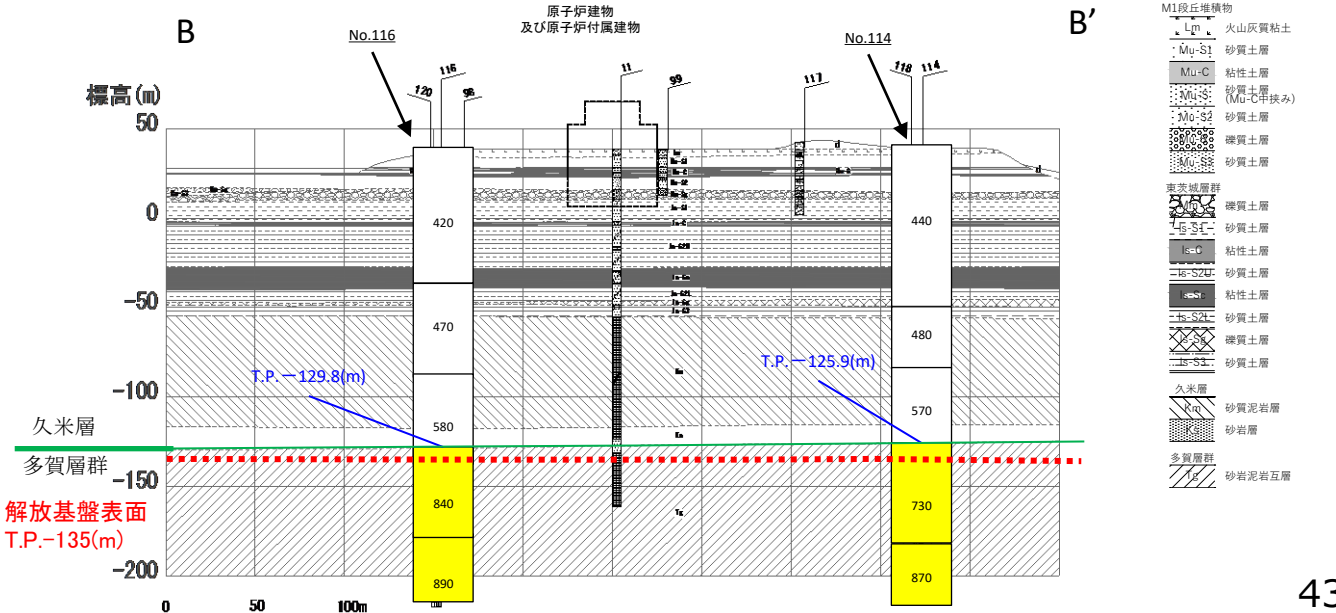
PS検層位置図
