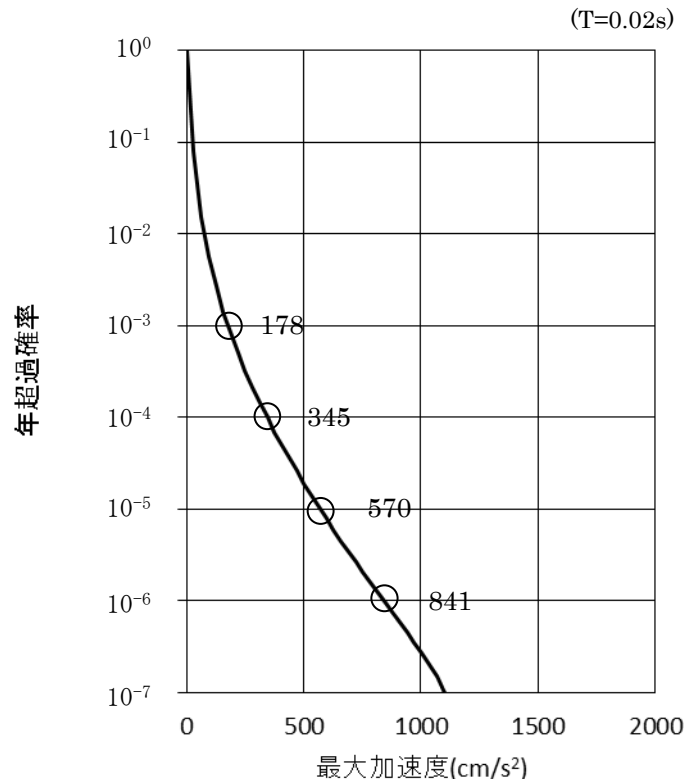
鉛直成分
