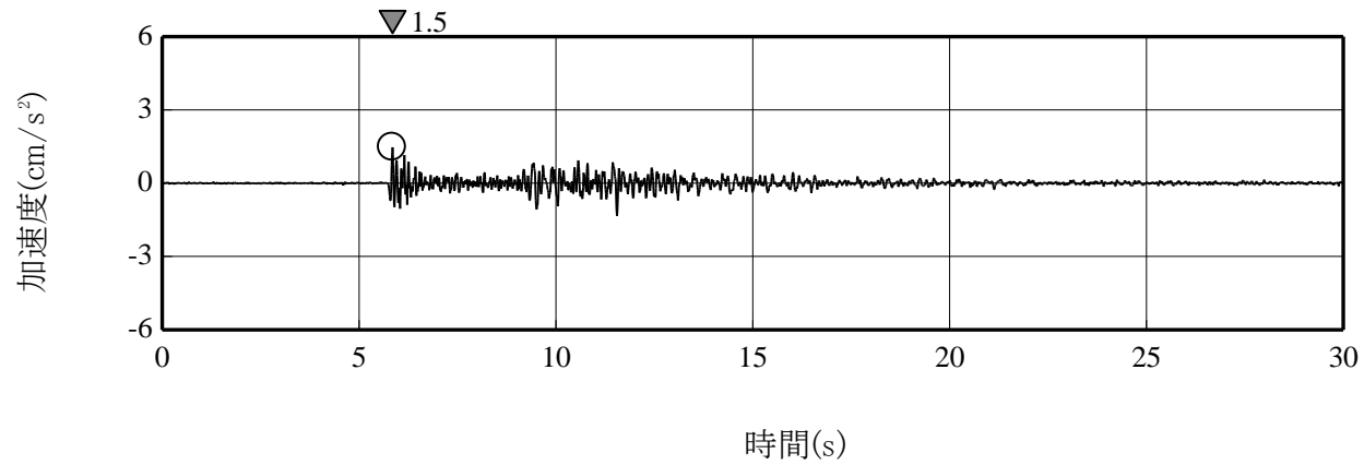
鉛直成分
