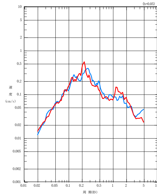
UD成分
