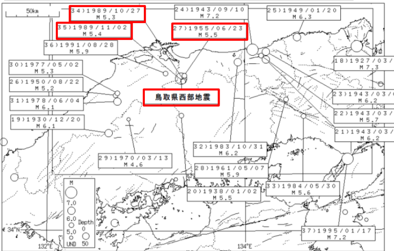
過去の被害地震(1926～2000年)(気象庁(2000)より抜粋)
