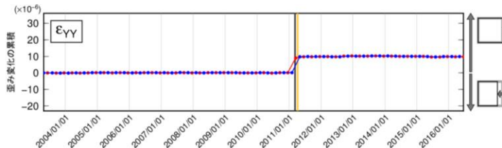
ひずみ変化の累積(大洗研敷地周辺)
