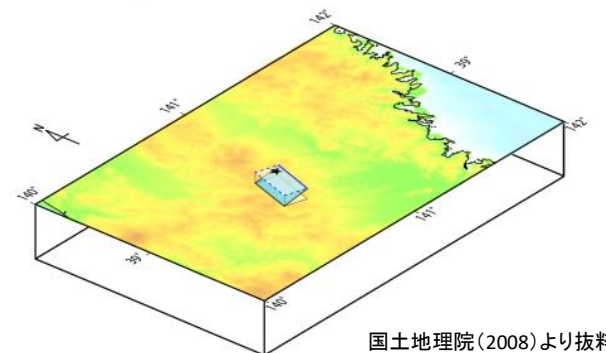
平成20年 (2008年) 岩手・宮城内陸地震の震源断層モデルの概念図
