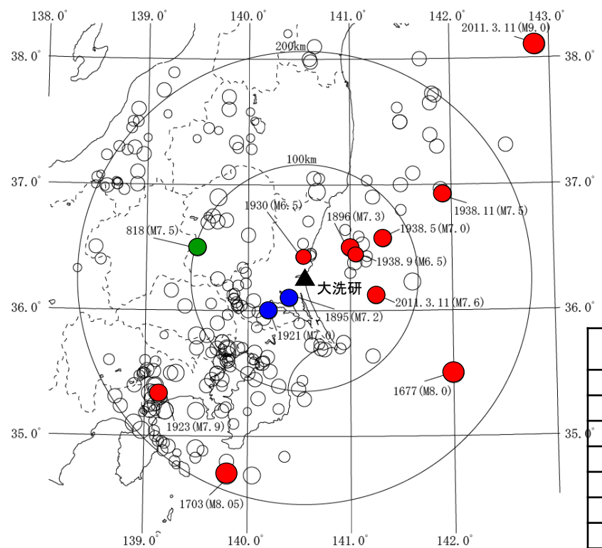
敷地周辺の被害地震の震央分布図 (日本被害地震総覧及び気象庁カタログ) ○ 敷地周辺で震度5弱程度以上と推定される地震 ● 内陸地殻内地震 ● プレート間地震 ● 海洋プレート内地震 ○ 8.0 ≤ M ○ 7.0 ≤ M < 8.0 ○ 6.0 ≤ M < 7.0 ○ 5.0 ≤ M < 6.0 ○ M < 5.0
