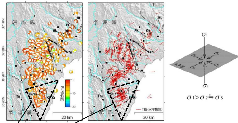
下図の三角形要素11を示す 図11 得られたメカニズム解とT軸の分布 左：下半球投影のメカニズム解。深さで色分けした。井戸沢断層(It)と湯ノ岳断層(Yn)の地表地震断層 (Mizoguchi et al. in preparation) を○で示す。中：メカニズム解のT軸方位 (水平投影)。右：推定される応力場の概念図。 青柳・上田(2012)に一部加筆
