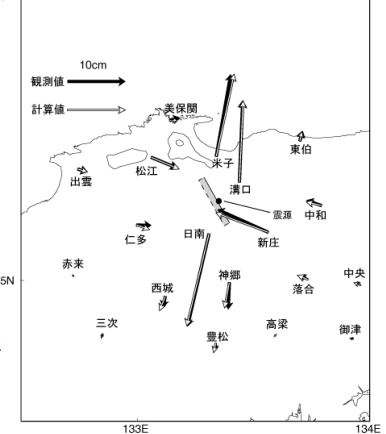
断層パラメーター 新発北西断層の位置：東経133度18分 北緯35度21分 上縁の深さ：1km 断層の大きさ：20km(長さ)×10km(幅) 走向：北から時計回りに152度 傾斜角：86度 すべり角：-7度 すべり量：-1.4m M 0 (モーメントマグニチュード)：6.6相当
