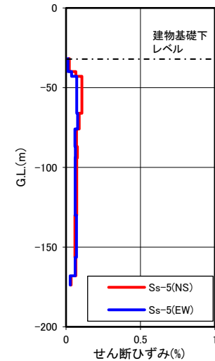
水平成分
