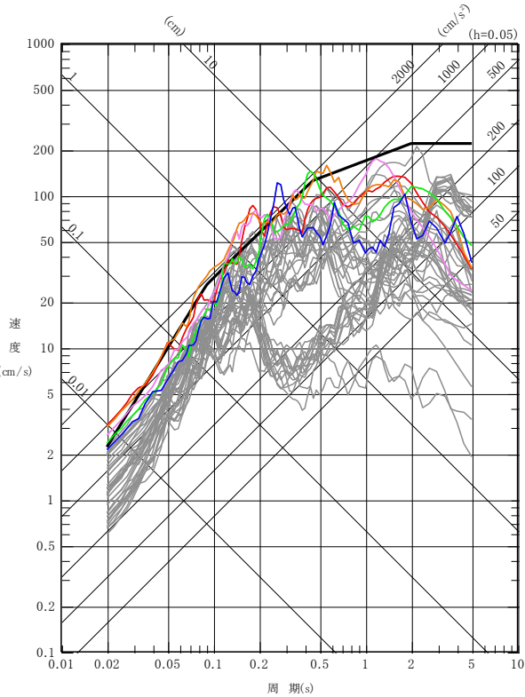
NS成分
