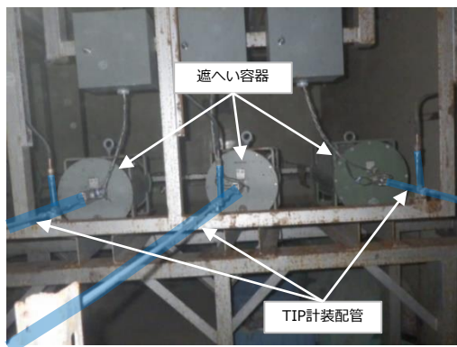
撤去対象の例：TIP計装配管，遮へい容器，機器サポート
