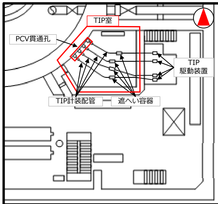
TIP計装配管等の配置 (3号機原子炉建屋1階 南東エリア)
