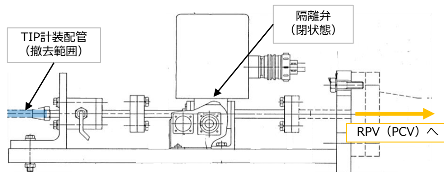
TIP計装配管とPCVの隔離状況
