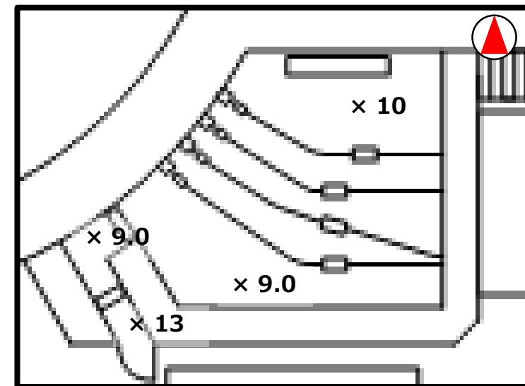
TIP室内の空間線量率（単位：mSv/h）
