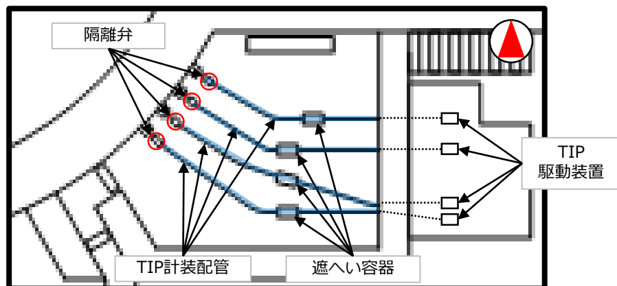
TIP室内の撤去対象（TIP計装配管，遮へい容器）の配置
