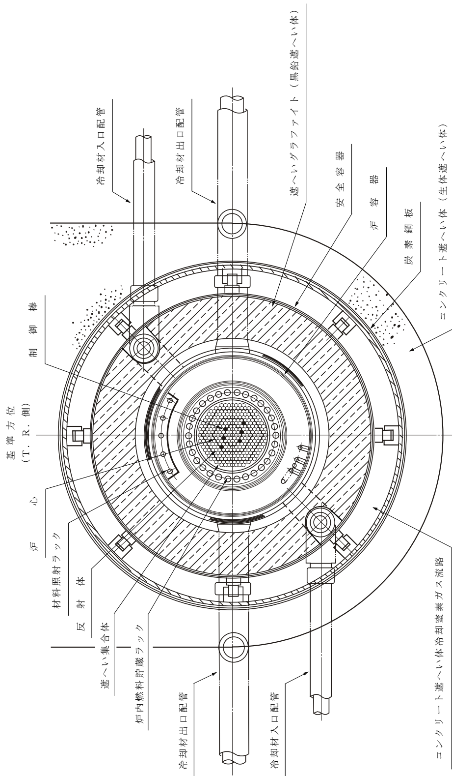
第 3.1.2 図 原子炉水平断面図
