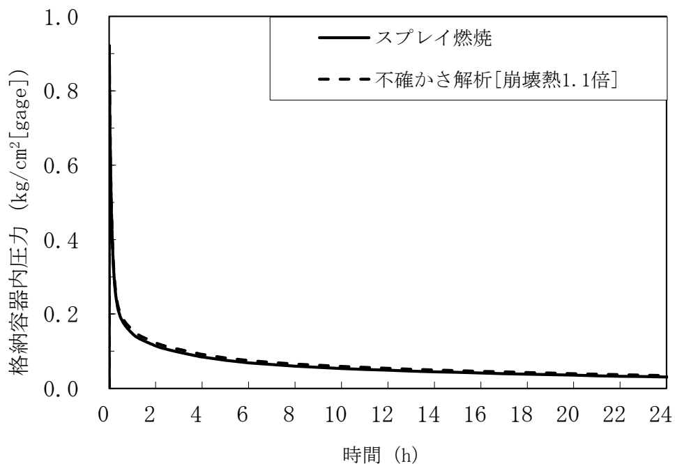
第 4.3.3.1.33 図 格納容器内圧力の推移 (不確かさの影響評価)
