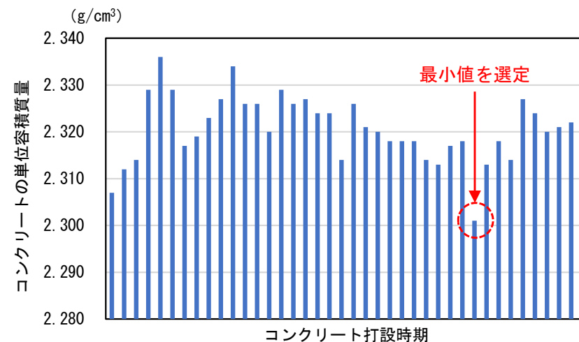
建設時のコンクリートの単位容積質量の事例 (川内1号炉 原子炉格納施設等 外部遮蔽壁)
