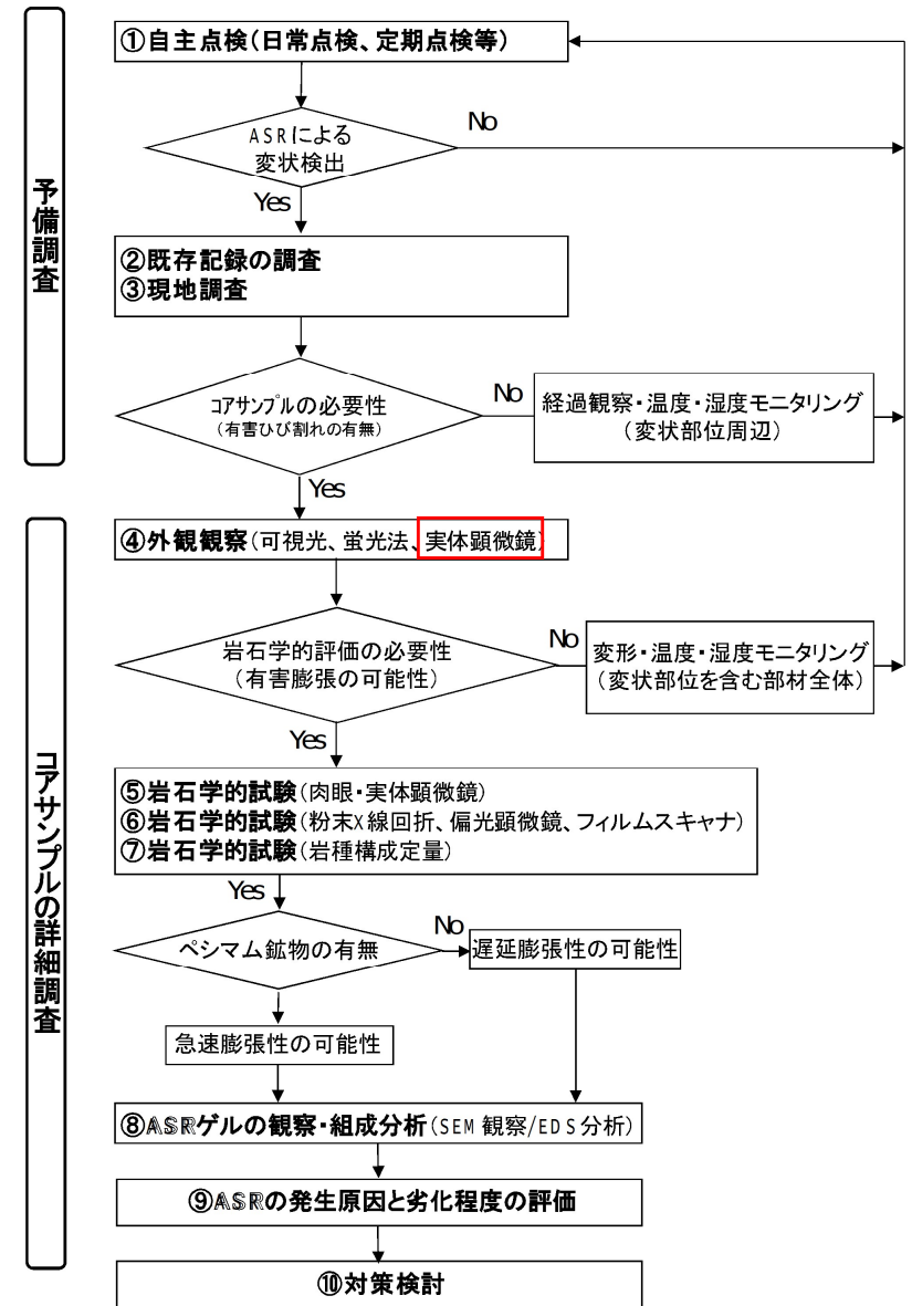
コンクリート構造物のASR診断フロー(例) (安全研究成果報告 運転期間延長認可制度及び高経年化対策制度に係る技術的知見の整備に関する研究(RREP-2018-1004)より)
