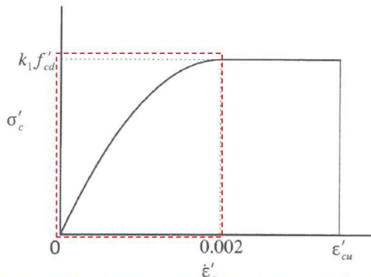
コンクリートの応力-ひずみ曲線
