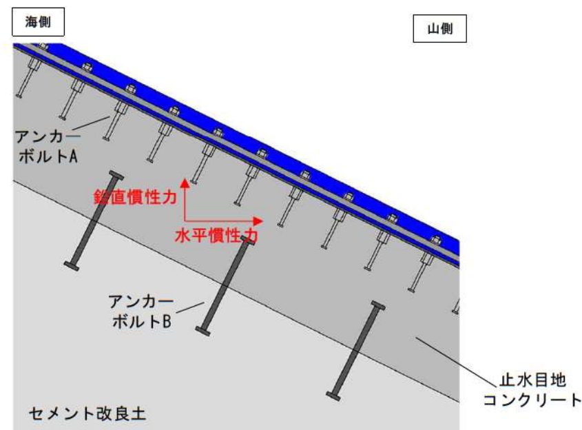
地震時にアンカーボルトBに生じる外力
