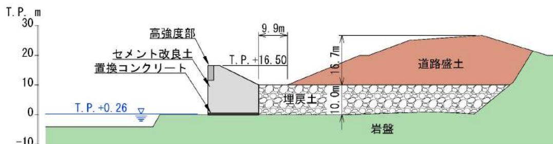
断面図(7-7')
