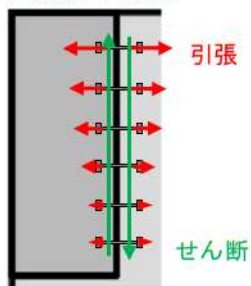
アンカーボルトの作用力 地震時
