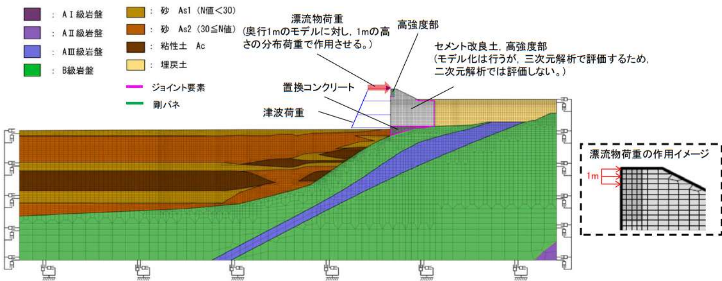
二次元動的FEM解析モデル図（津波時）
