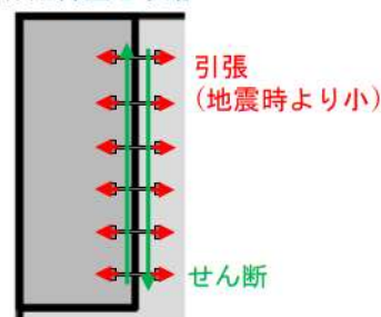
アンカーボルトの作用力 重畳時
