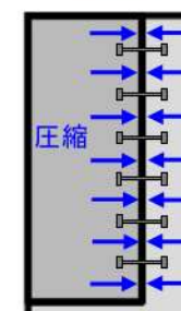
アンカーボルトの作用力 津波時
