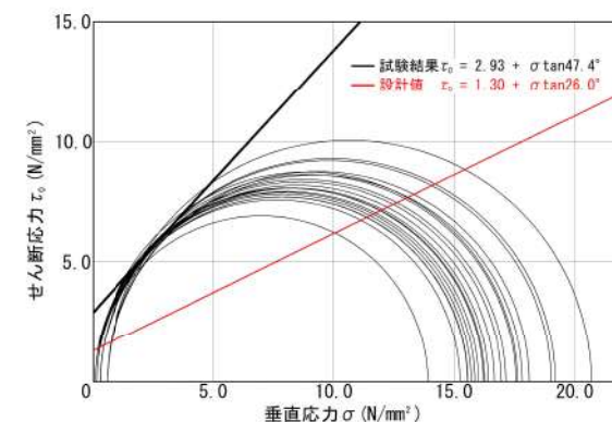
健全強度
