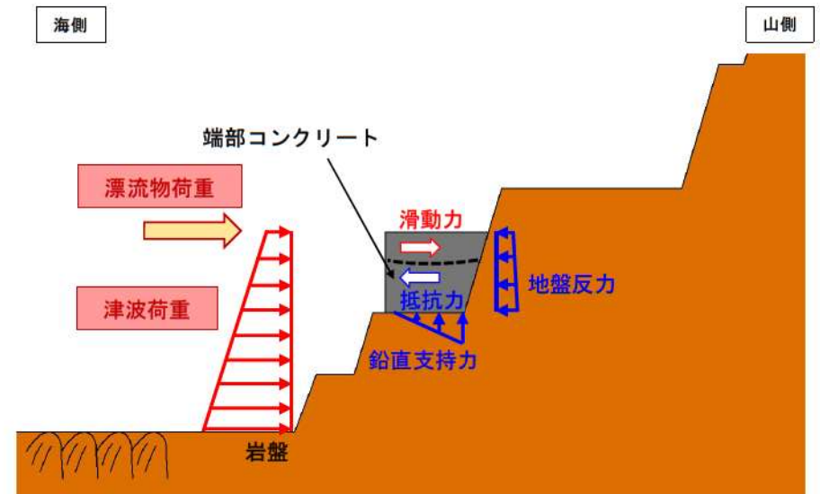
荷重図
