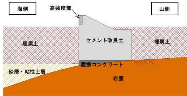
断面図 泊発電所
