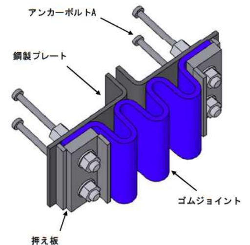
ゴムジョイント固定イメージ図
