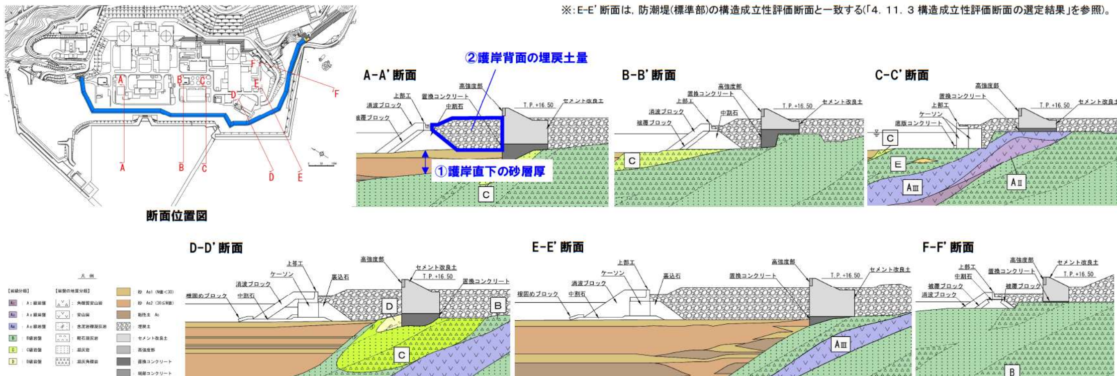
地質断面図
