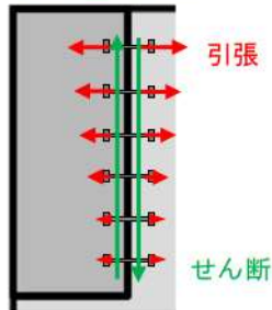
アンカーボルトの作用力
