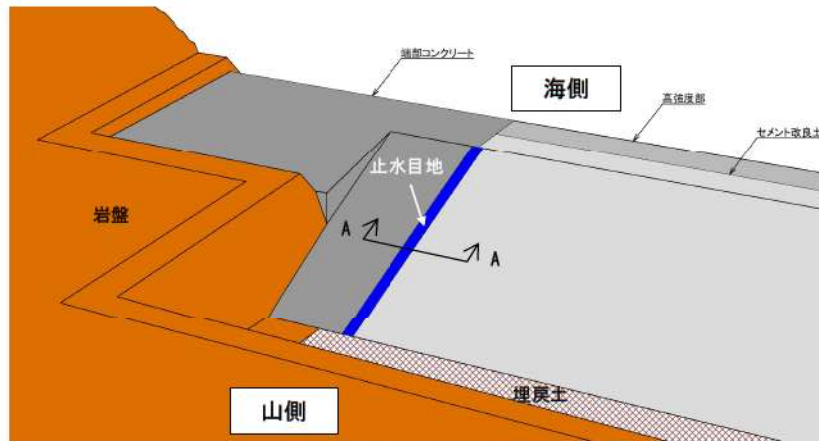
構造境界部の概要
