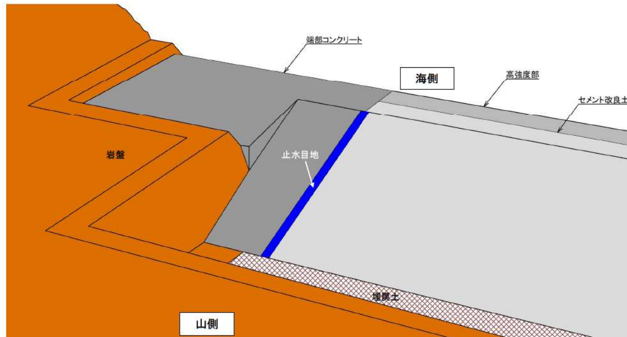
構造境界部の概要
