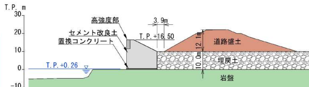
断面図(7a-7a')
