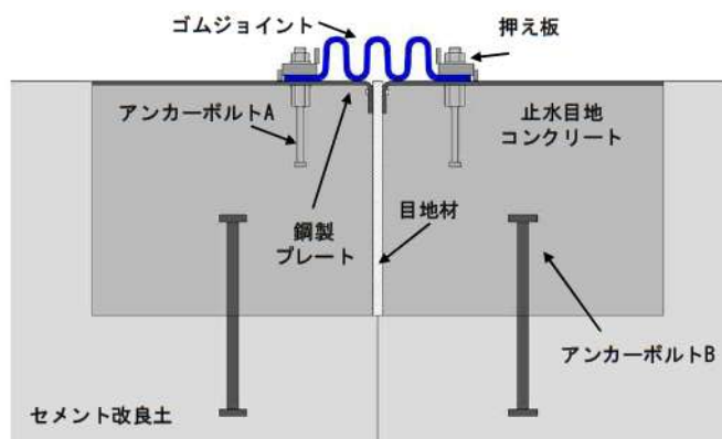
止水目地設置概要
