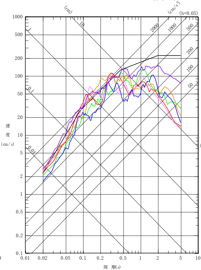
EW成分
