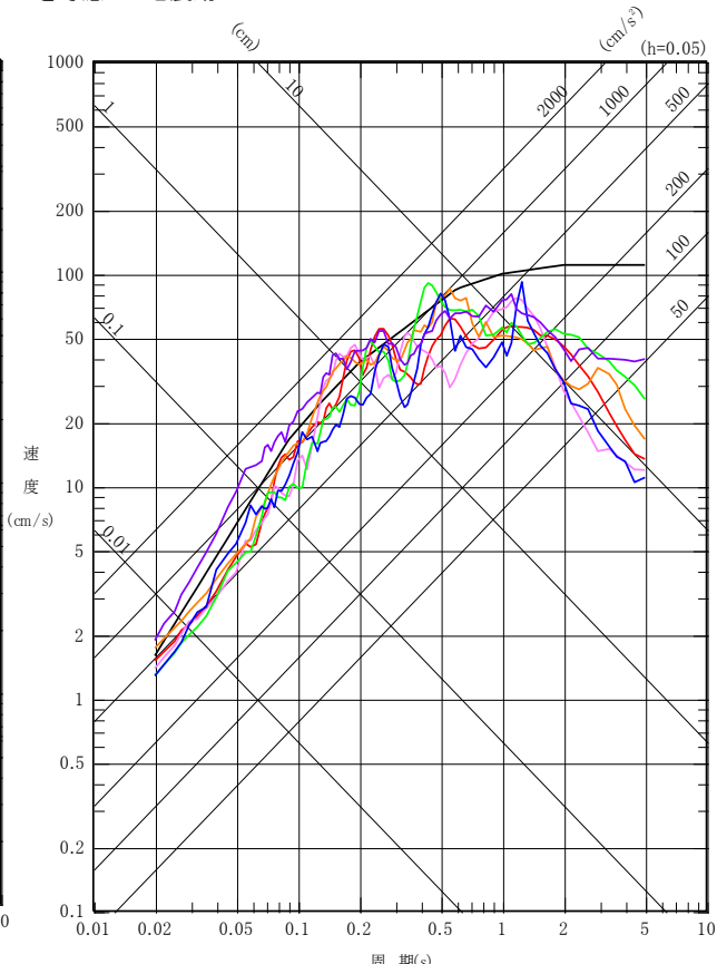
UD成分
