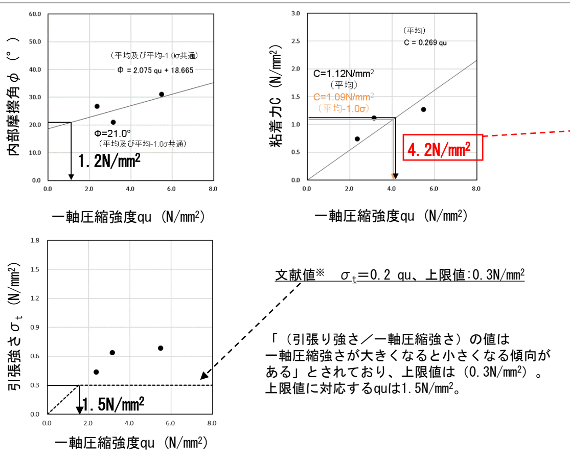
図1 室内配合試験による一軸圧縮強度 q_u と評価に用いる強度特性の相関関係(Mu-S 2 層) (内部摩擦角 \phi 、粘着力C、引張強さ \sigma_t )
