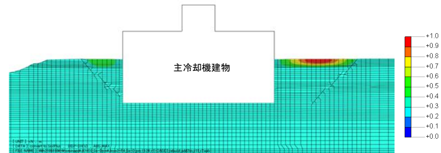
最大変位(水平成分)(m)
