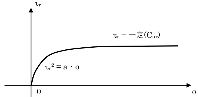
残留強度 \tau_r
