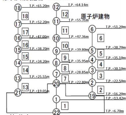
基礎底面 ○:質点番号 □:部材番号
