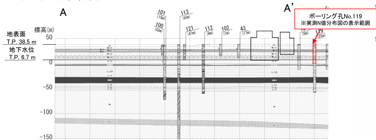
地質断面図(A-A'断面)
