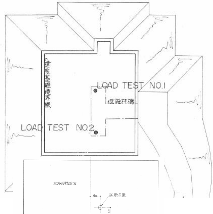
原子炉建物及び原子炉附属建物、主冷却機建物 地耐力検査位置
