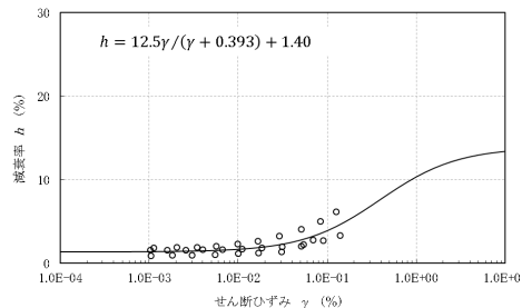
減衰率 h
