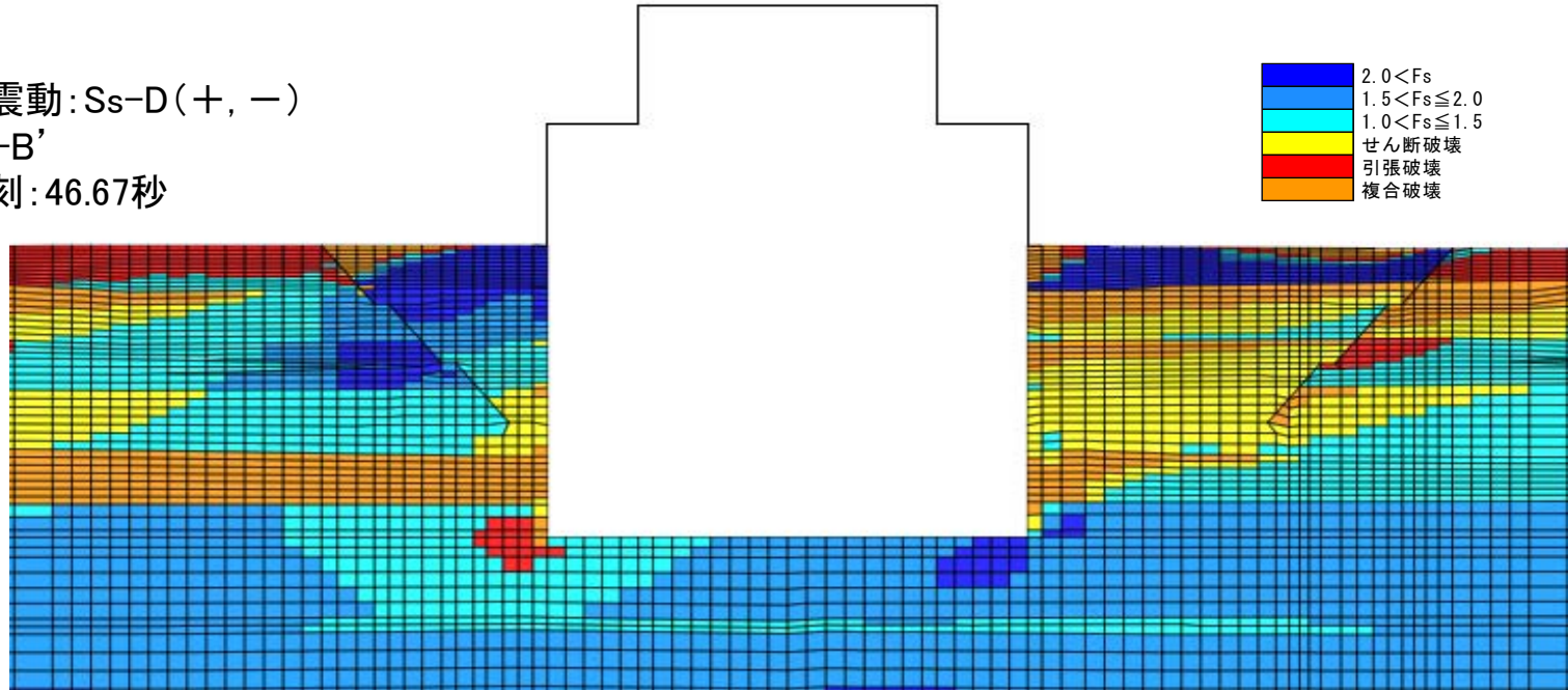
局所安全率
