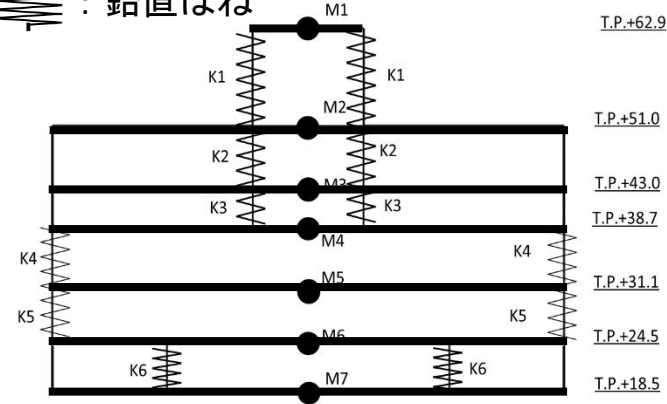
基礎底面 有限要素モデル (水平・鉛直同時加振モデル)
