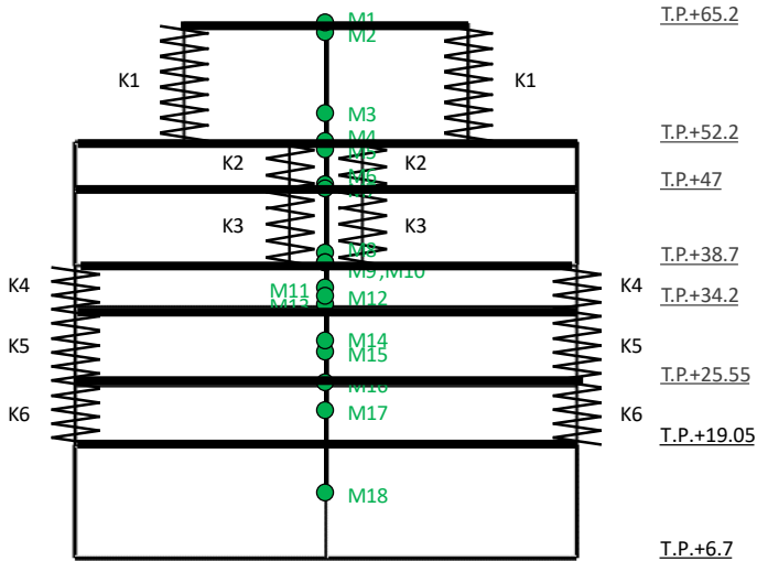
有限要素モデル
