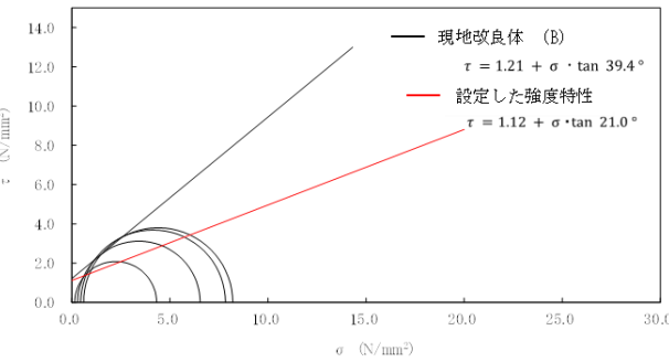
現地改良体 B (埋戻土)
