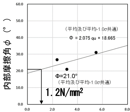
一軸圧縮強度 q_u (N/mm 2 )
