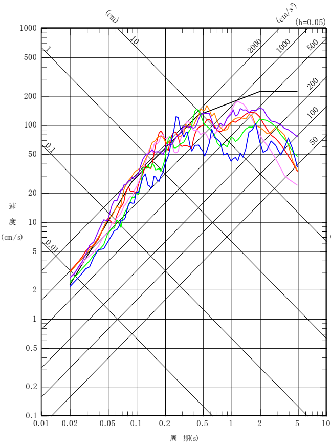
NS成分
