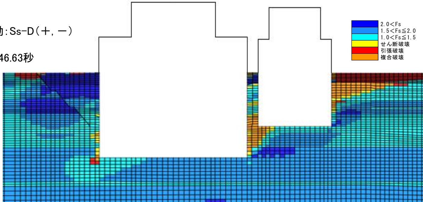
局所安全率
