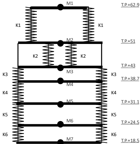
有限要素モデル
