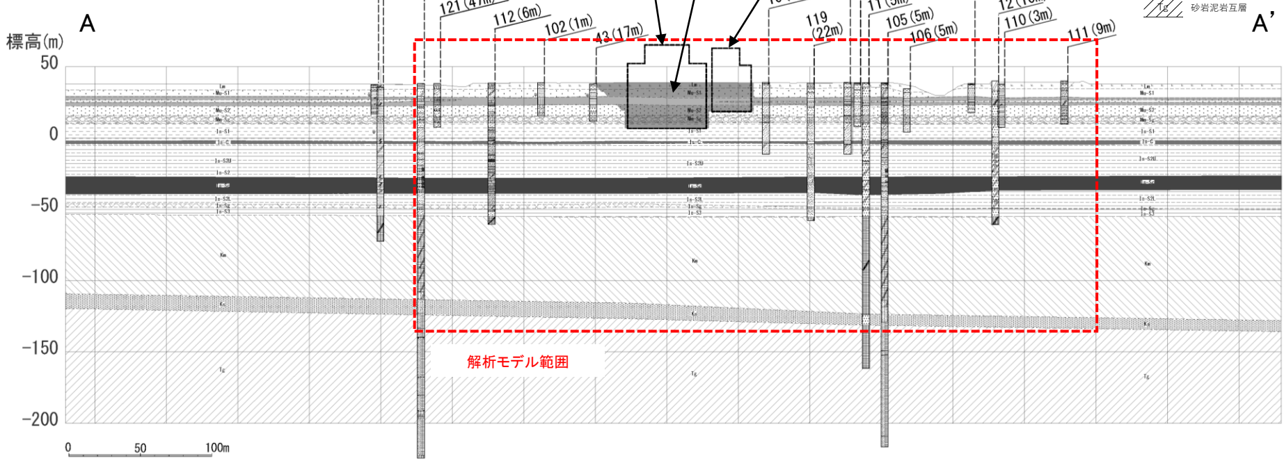
A-A'断面(南北方向)
