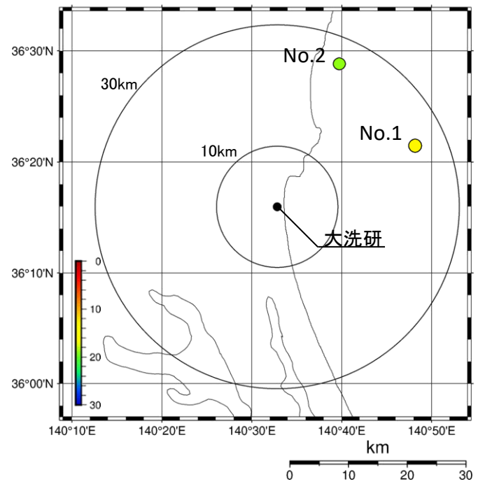
震央分布図
