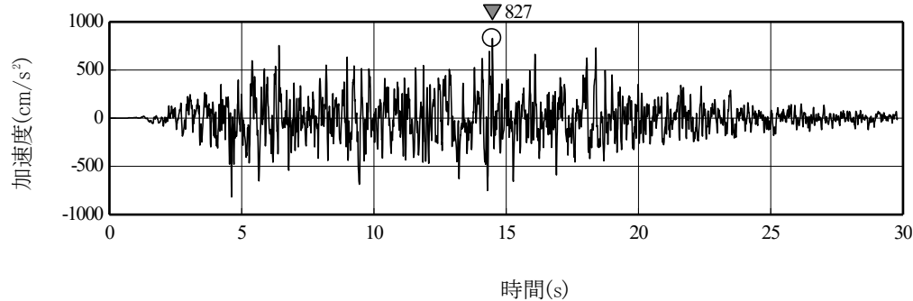
水平成分
