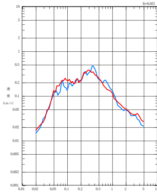
EW成分
