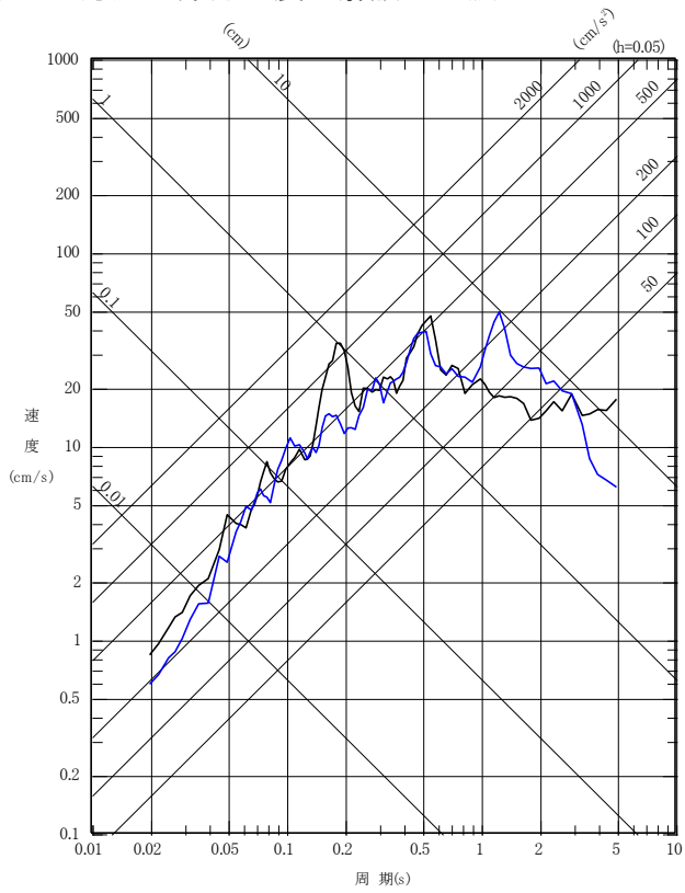
UD成分
