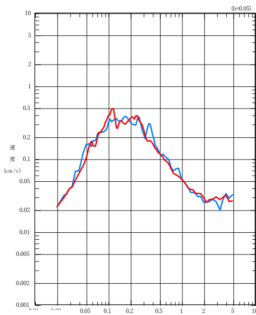
NS成分
