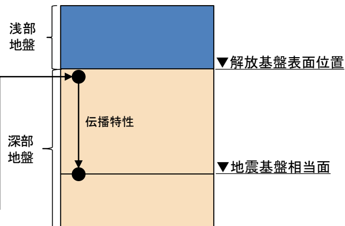
解放基盤表面位置から地震基盤相当面までの引戻しのイメージ
