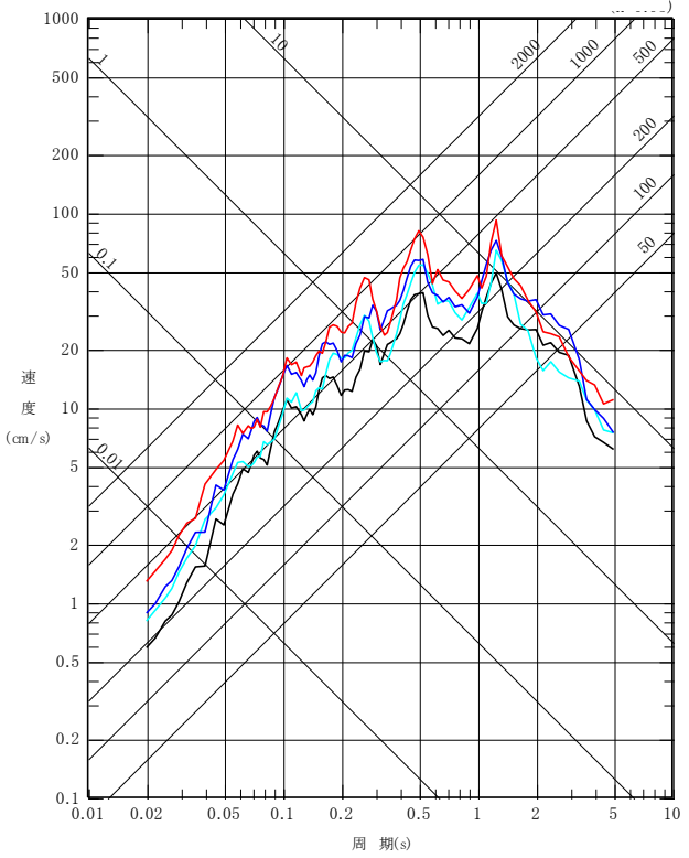
UD成分
