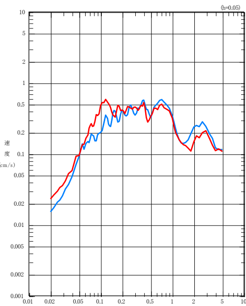
NS成分
