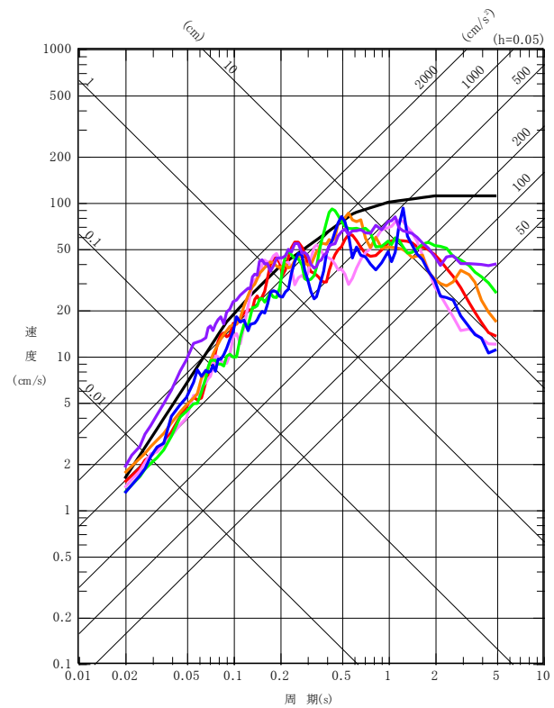
UD成分
