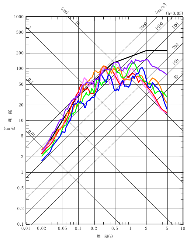
EW成分
