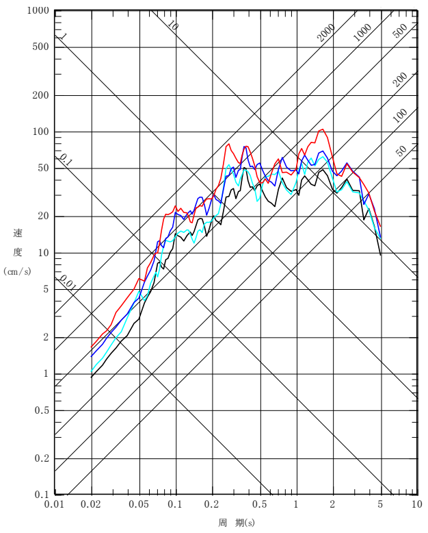
EW成分
