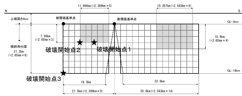
断層傾斜角の不確かさを考慮した震源モデル
