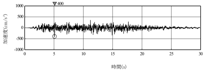
鉛直成分
