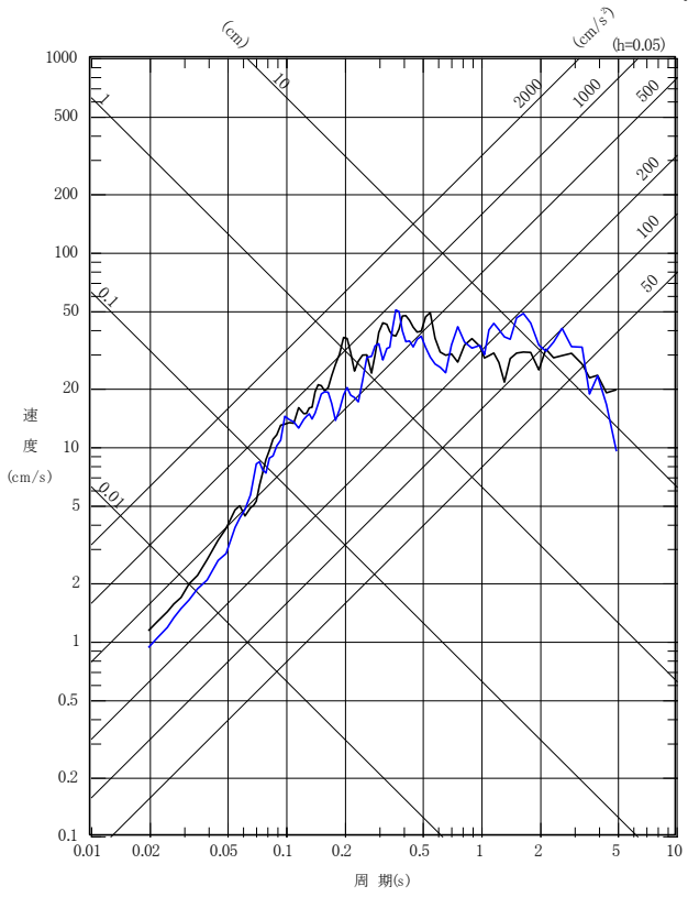
EW成分
