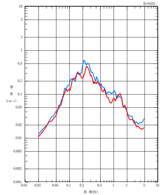
UD成分
