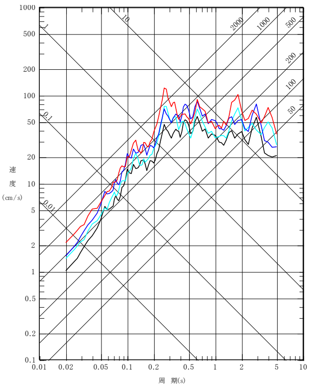
NS成分
