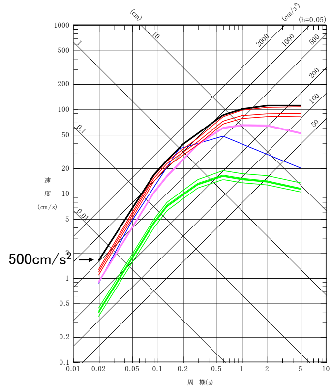
鉛直成分
