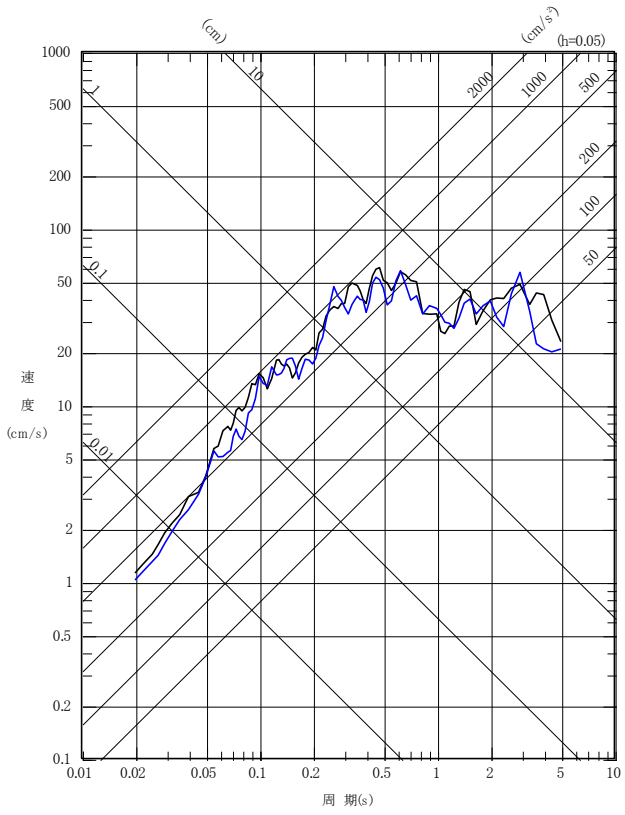
NS成分
