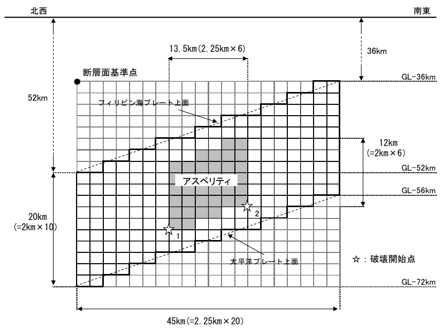
震源モデル
