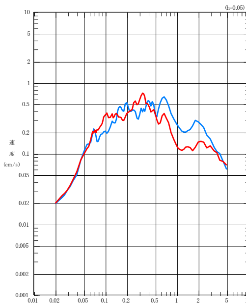
EW成分
