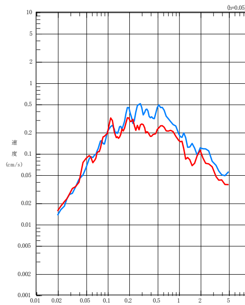
UD成分
