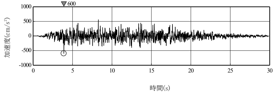
水平成分
