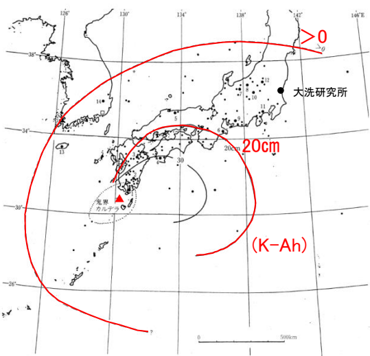
図 2.1-2 鬼界アカホヤテフラ (K-Ah) の等層厚線図と主な産出地点。点線内は火砕流堆積物 (K-Ky) の分布範囲を示す。
