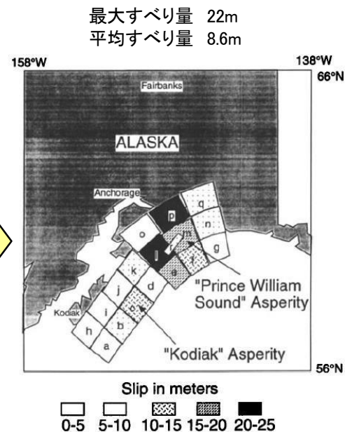
【地震時すべり量(1964年)(a)】
