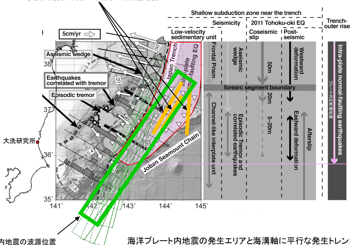
海溝軸(南側・北側)に平行な正断層型地震のトレンド
