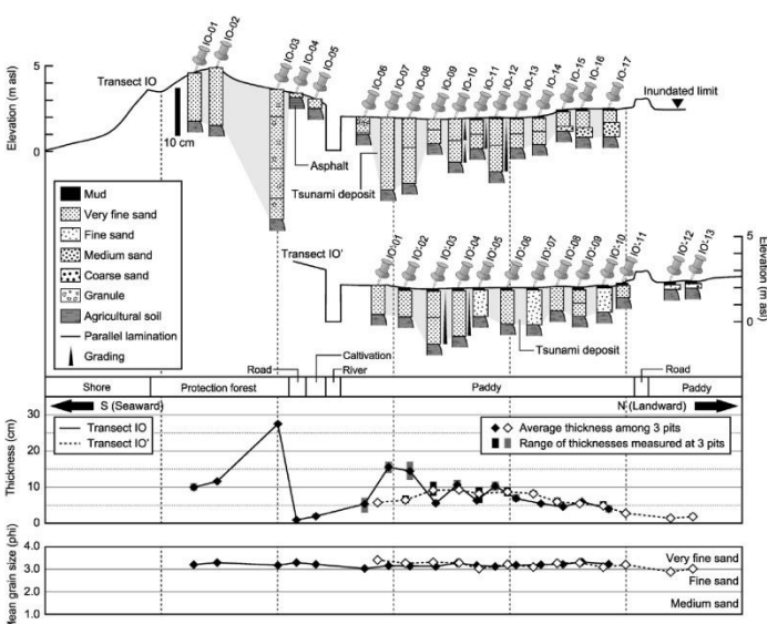
鹿島港(上)及び飯岡(下)における測線内の地形断面、柱状図、及び層厚変化(山田・藤野(2013))
