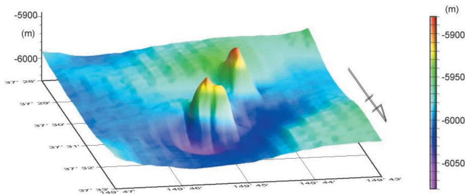
図4 北北東から眺めた2つのプチスポット火山の鳥瞰図。山体の規模は、いずれも長径1 km、比高100~200 m程度である。調査船による音波を用いた海底地形探査でやっと初めてその存在が明らかとなる大きさである。緯度経度を示すグリッドは1分がおおよそ1.85 kmに相当。図2の幅幅が約1100 kmであるのに対し、この図の幅幅はたった7.4 kmに過ぎないことに注意。
