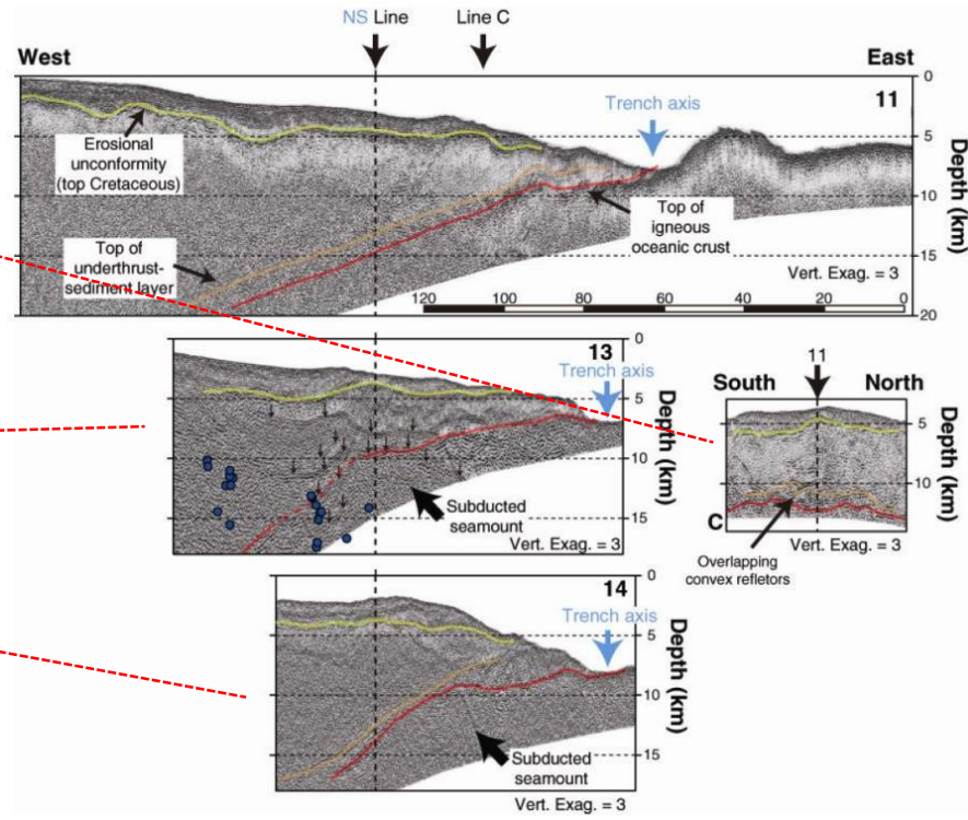
各測線における反射断面 (Mochizuki et al. (2008)に加筆)
