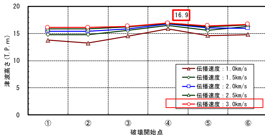
敷地前面海岸での津波高さ：(B-3：南へ10km移動)、破壊開始点及び破壊伝播速度のパラメータスタディ
