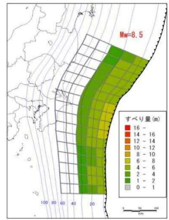
延宝房総沖地震(Mw 8.5)
