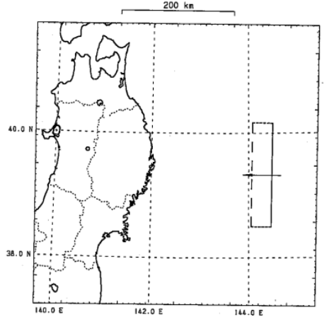
昭和三陸地震(Mw 8.1)
