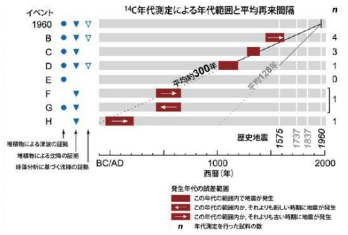
第2図 Maullinにおいて観察される津波堆積物とその履歴。Cisternas et al. (2005) 3) に基づく。 Figure 2. Tsunami deposit observed in Maullin and its history. Based on Cisternas et al. (2005).
