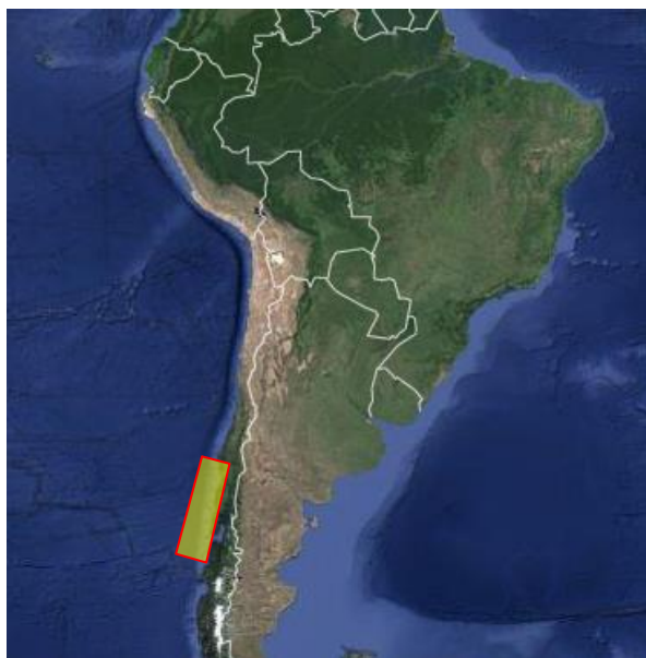
発生位置(1960年チリ地震)
