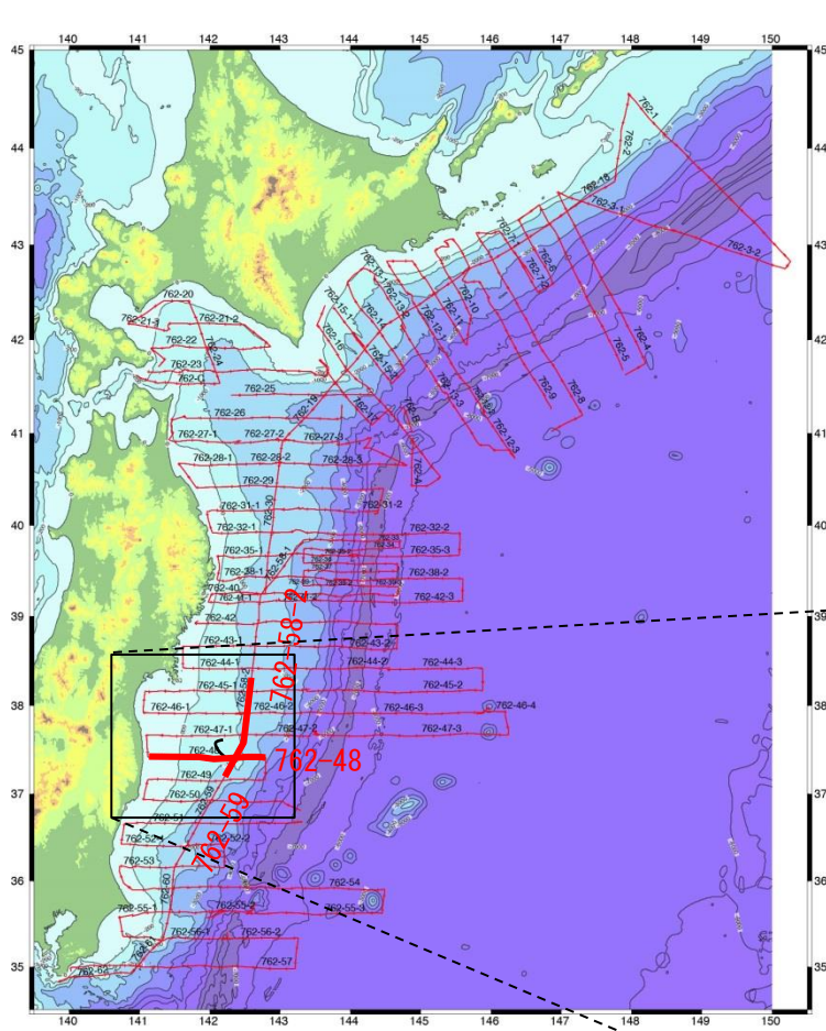
徳山他(2011)に示されている海底地すべり
