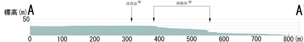
A-A' 断面図
