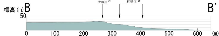
B-B' 断面図
