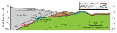
茨城県沖のプレート境界付近の地質構造 (Moore et al. (2015))
