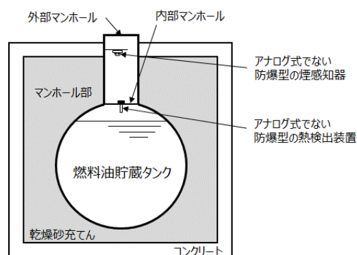
第 3-2-5 図 □の火災感知器配置図（断面図）
