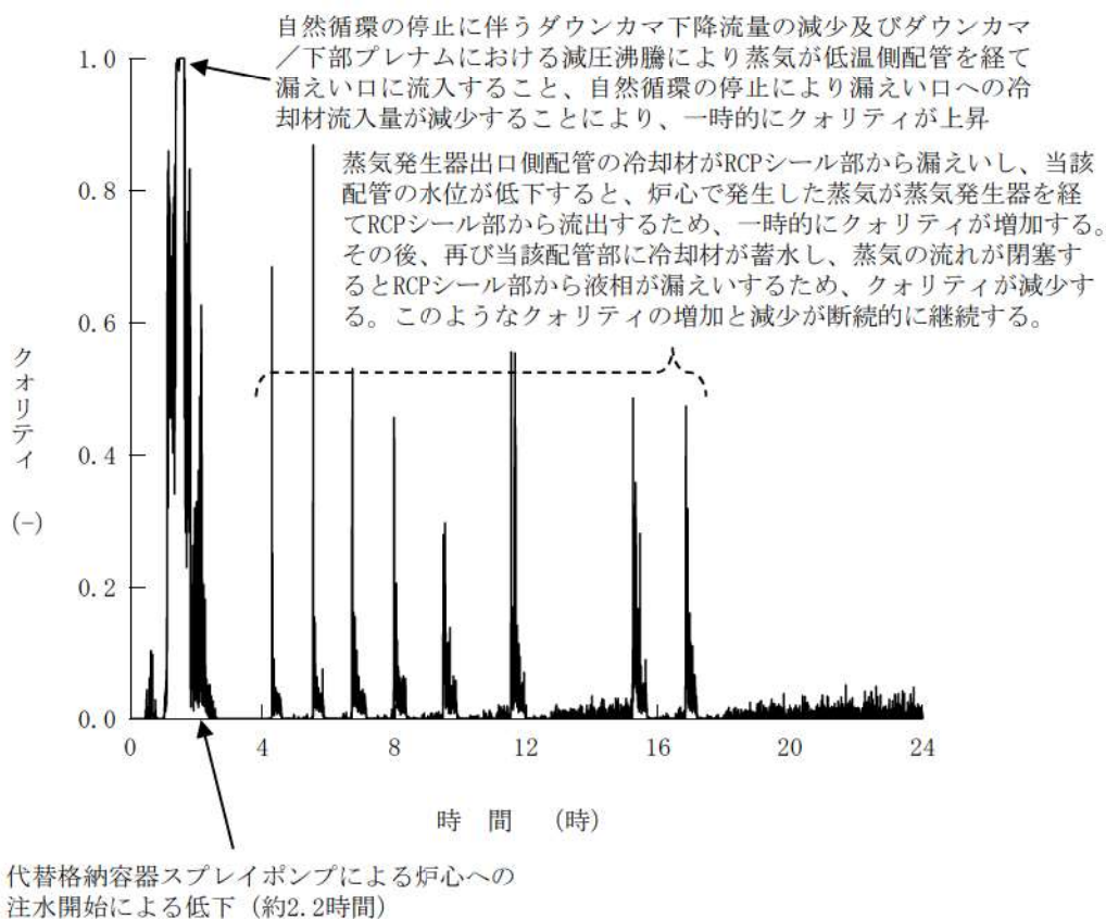
第 7.1.2.11 図 RCP シール部からの漏えいのクオリティの推移 (RCP シール LOCA が発生する場合)
