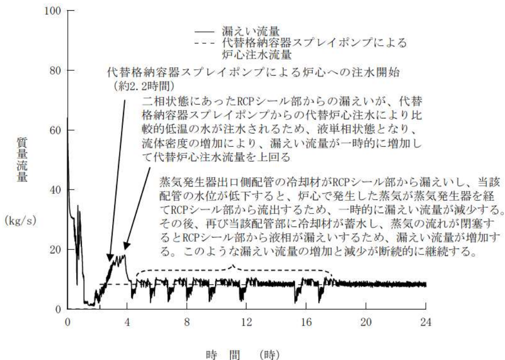
第 7.1.2.10 図 漏えい流量と注水流量の推移 (RCP シール LOCA が発生する場合)
