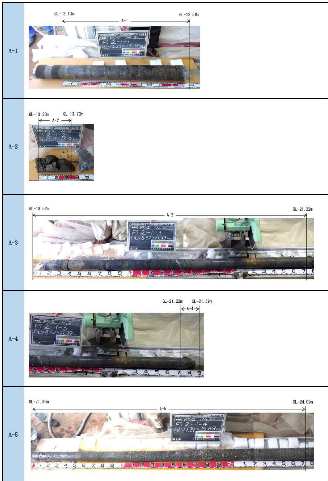
参考 1-34 図 (3/10) ボーリング柱状図・コア写真 (FS-2)
