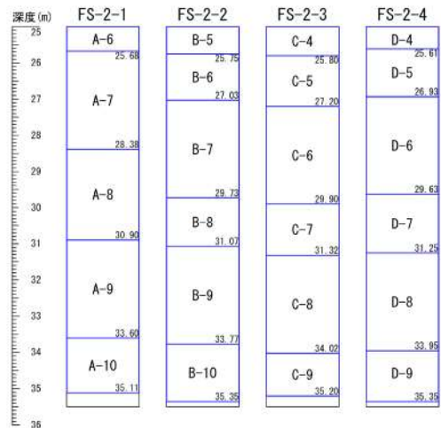
参考 1-34 図 (2/10) ボーリング柱状図・コア写真 (FS-2)
