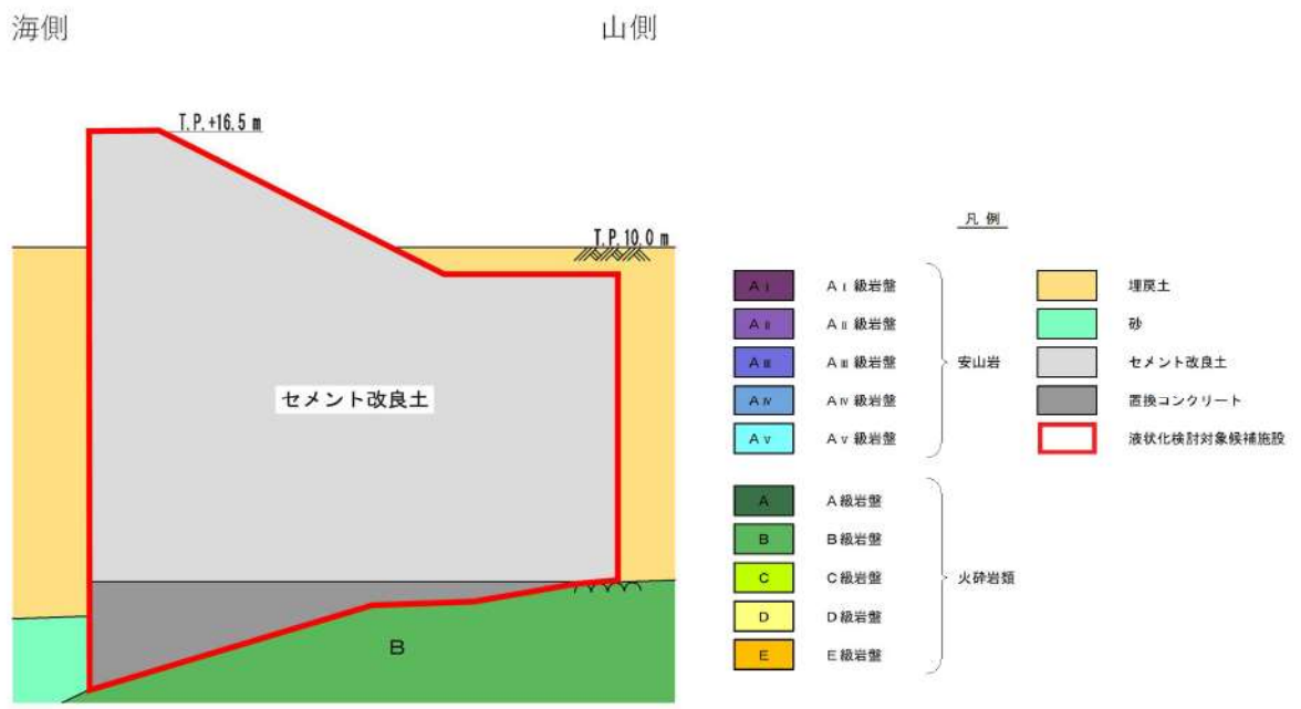
第 3.2-13 図 防潮堤断面図
