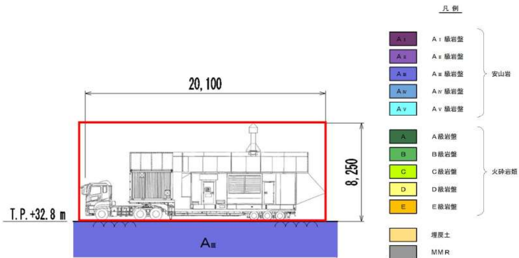
第 3.2-18 図 代替非常用発電機設置位置断面図
