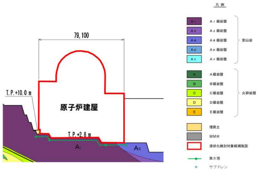
第 3.2-2 図 原子炉建屋断面図(南北)
