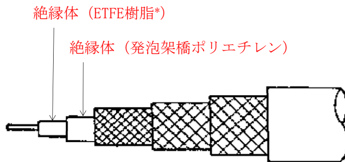
図 2.3-3 難燃三重同軸ケーブル（絶縁体が ETFE 樹脂*，発泡架橋ポリエチレン）の 絶縁部位 *：エチレン・四フッ化エチレン共重合樹脂
