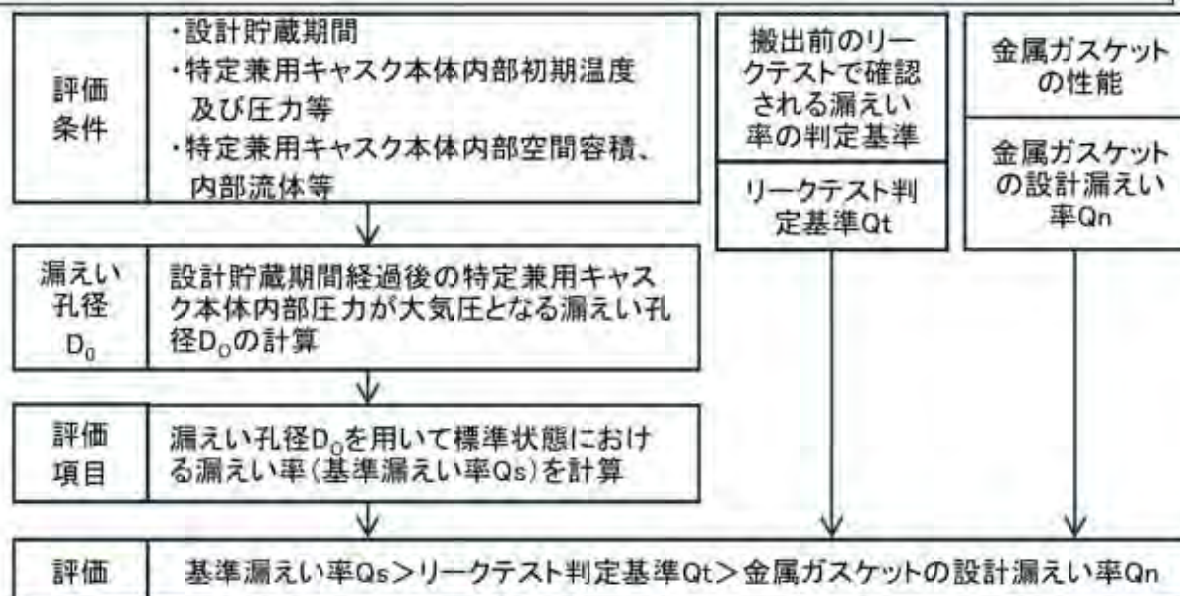
(閉じ込め機能評価フロー)
