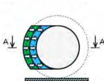
津波荷重の作用位置
