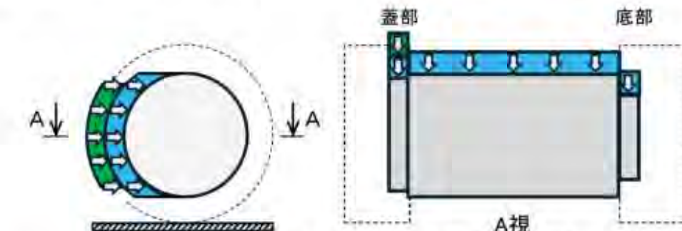
(2) MSF-24P(S)型の径方向衝突時
