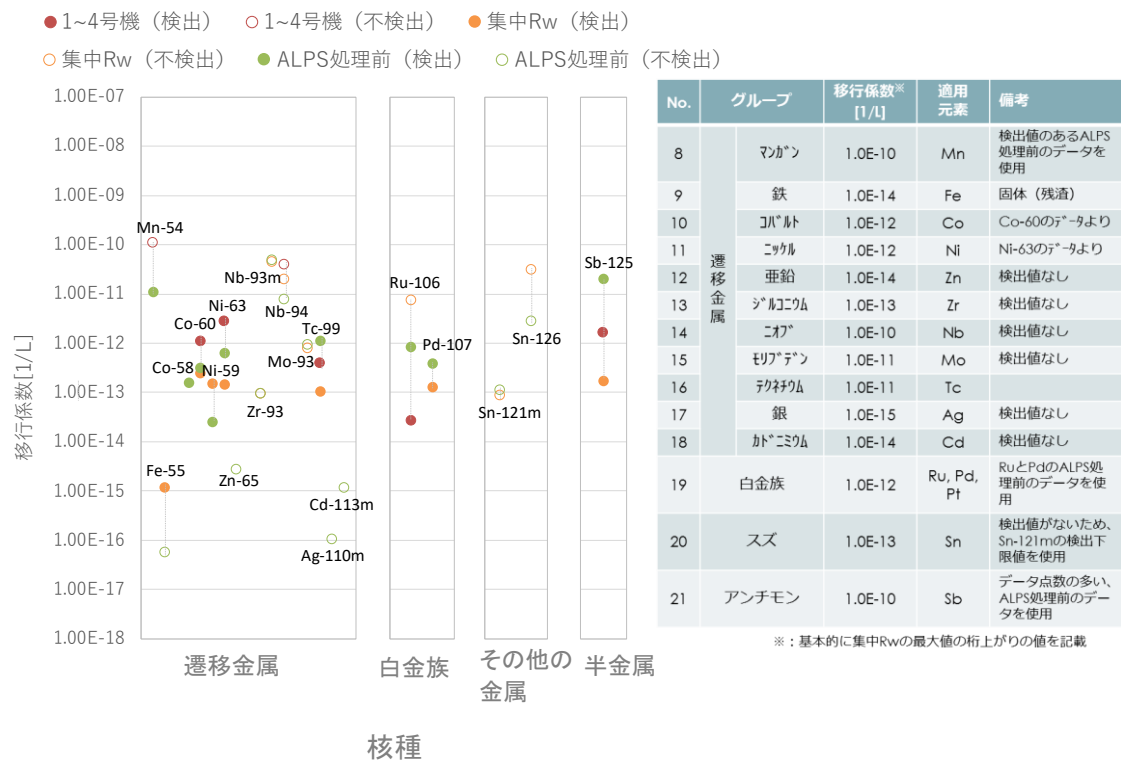
図 1.1.4-6 移行係数 (2/3)
