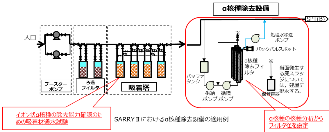
図 1.1.4-7 α核種除去設備の適用例
