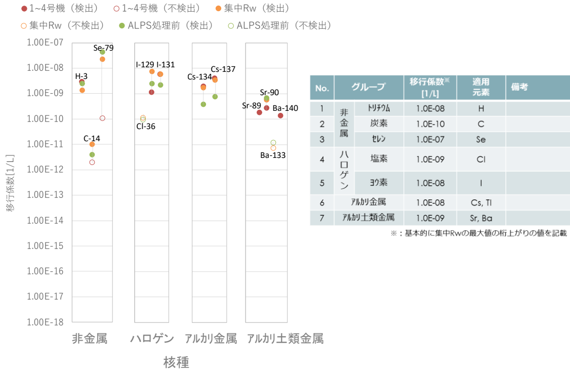
図 1.1.4-6 移行係数 (1/3)
