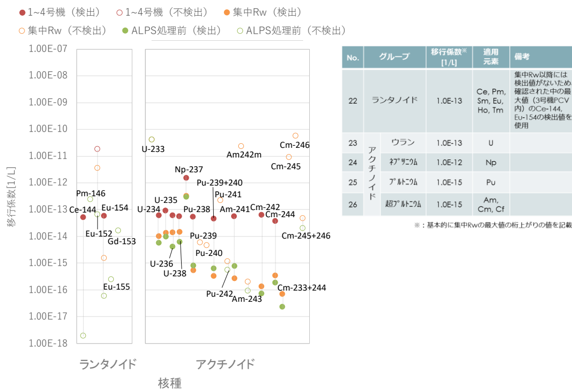
図 1.1.4-6 移行係数 (3/3)
