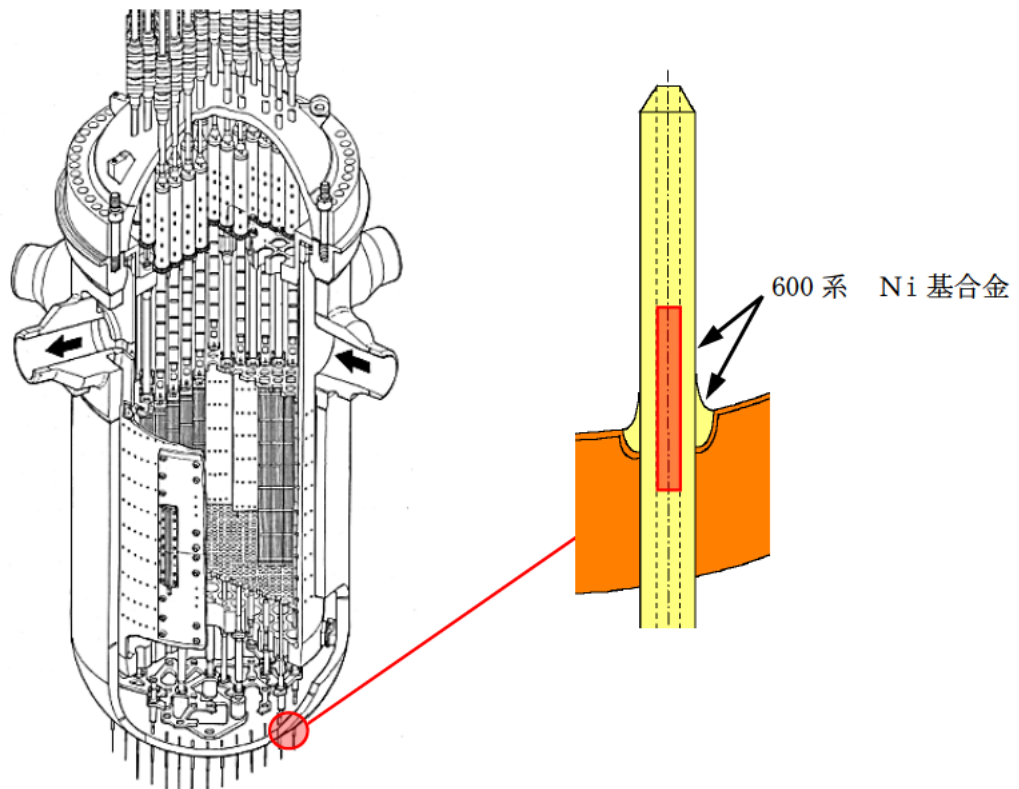
図3.3.1.2 試験対象 (BMI)
