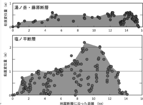
図2 塩ノ平地断層および湯ノ岳・藤原断層に沿って出現した地震断層の鉛直変位量分布
