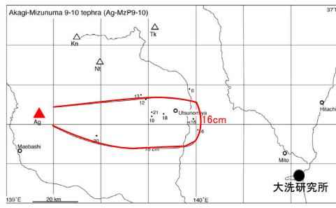
第23図 赤城水沼9-10テフラ(Ag-MzP9-10)の分布
