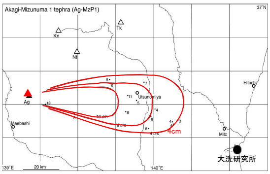
第19図 赤城水沼1テフラ(Ag-MzP1)の分布 数字は降下火砕堆積物の層厚で、単位はcm。Ag = 赤城火山；Hu = 嬖ヶ岳火山；Kn = 鬼怒沼火山；Nr = 男体火山；Tk = 高原火山。
