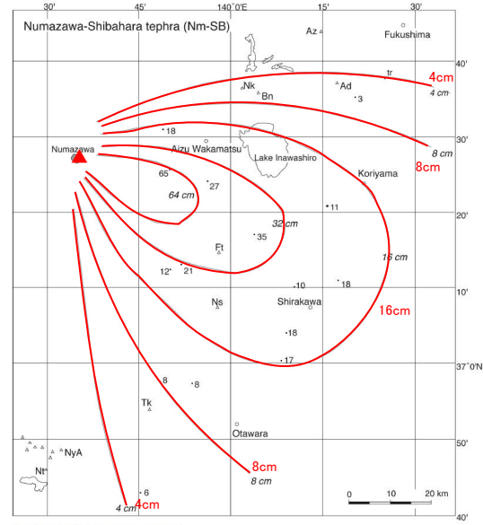
第28図 沼沢芝原テフラ (Nm-SB) の分布。 数字は降下火砕堆積物の層厚で、単位は cm。Ad = 安達太良火山; Ae = 吾妻火山; Bn = 磐梯火山; Ft = 二岐山火山; Kk = 黒鷹火山; Nm = 沼沢火山; Ns = 那須火山群; Nt = 男体火山; NyA = 女峰赤塚火山; Tk = 高原火山。山元 (2003) を一部改変。
