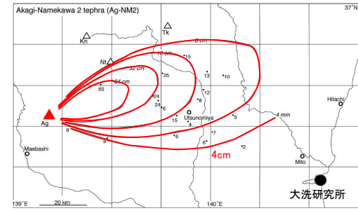
第18図 赤城行川2テフラ(Ag-NM2)の分布 数字は降下火砕堆積物の層厚で、単位はcm。Ag = 赤城火山；Hu = 嬖ヶ岳火山；Kn = 鬼怒沼火山；Nr = 男体火山；Tk = 高原火山。
