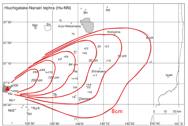
第35図 燧ヶ岳七入テフラ (Hu-NN) の分布。 数字は降下火砕堆積物の層厚で、単位は cm。Ad = 安達太良火山; Bn = 磐梯火山; Ft = 二岐山火山; Hu = 燧ヶ岳火山; Kn = 鬼怒沼火山; NKS = 日光白根火山; Nm = 沼沢火山群; Nt = 男 体火山; NyA = 女峰赤塚火山; Sn = 砂小原カルデラ; Tk = 高原火山。山元 (1999b) を一部改変。
