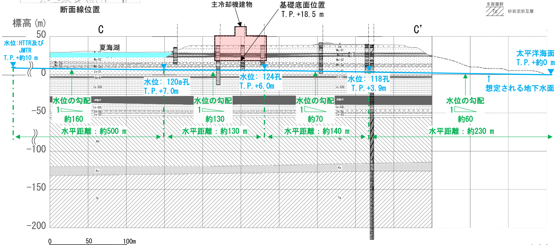
C-C' 断面(東西方向)
