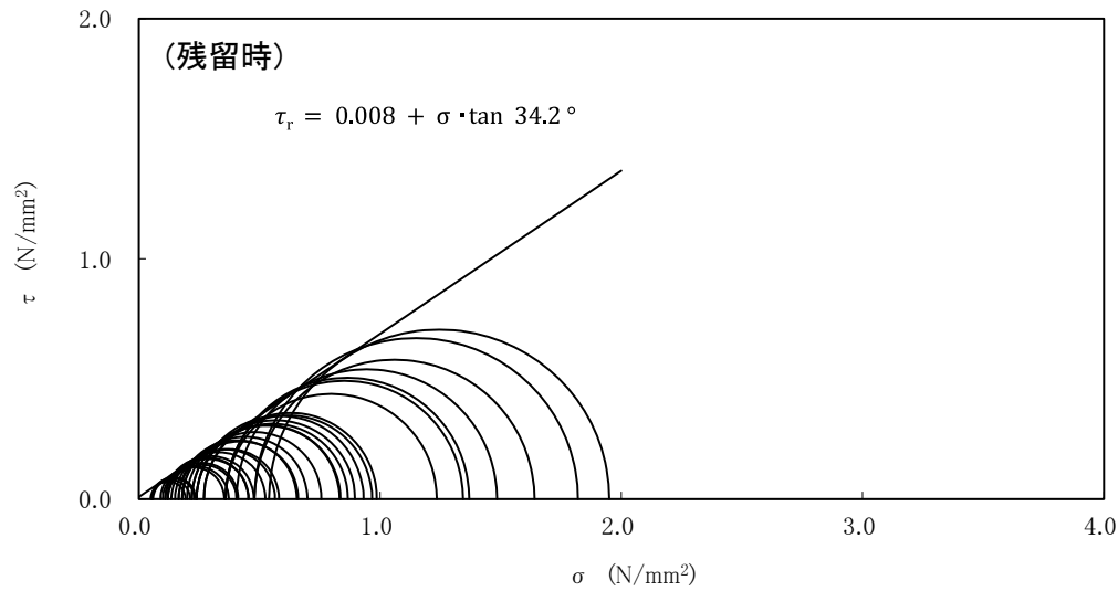
強度特性(埋戻土)
