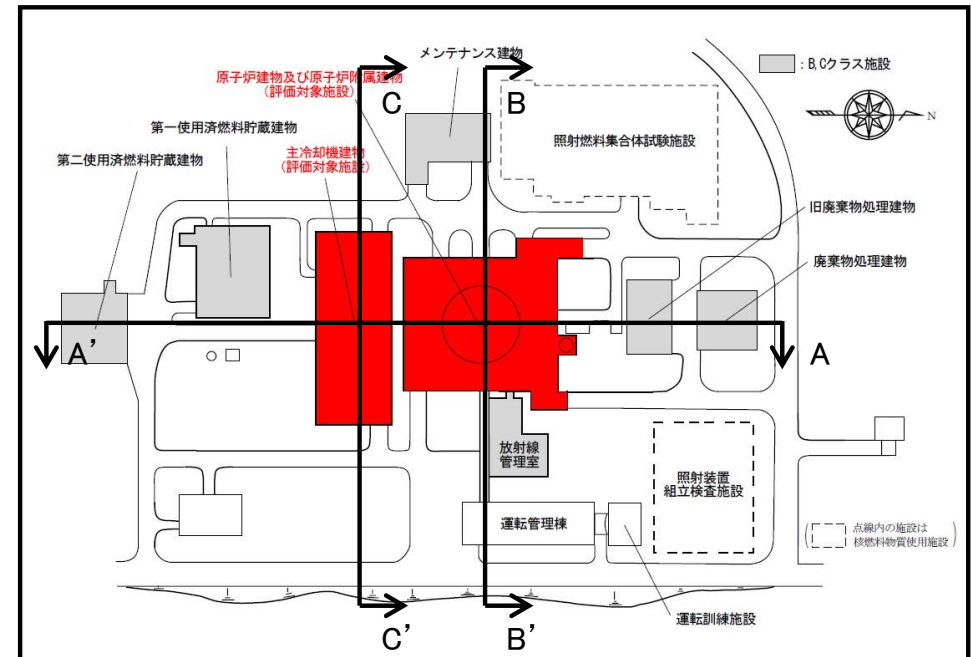
評価対象施設配置図
