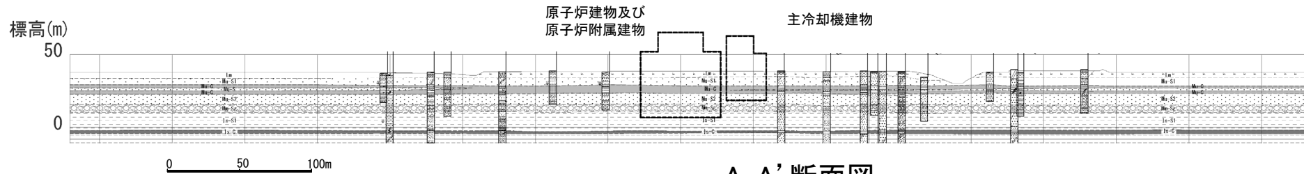
A-A' 断面図
