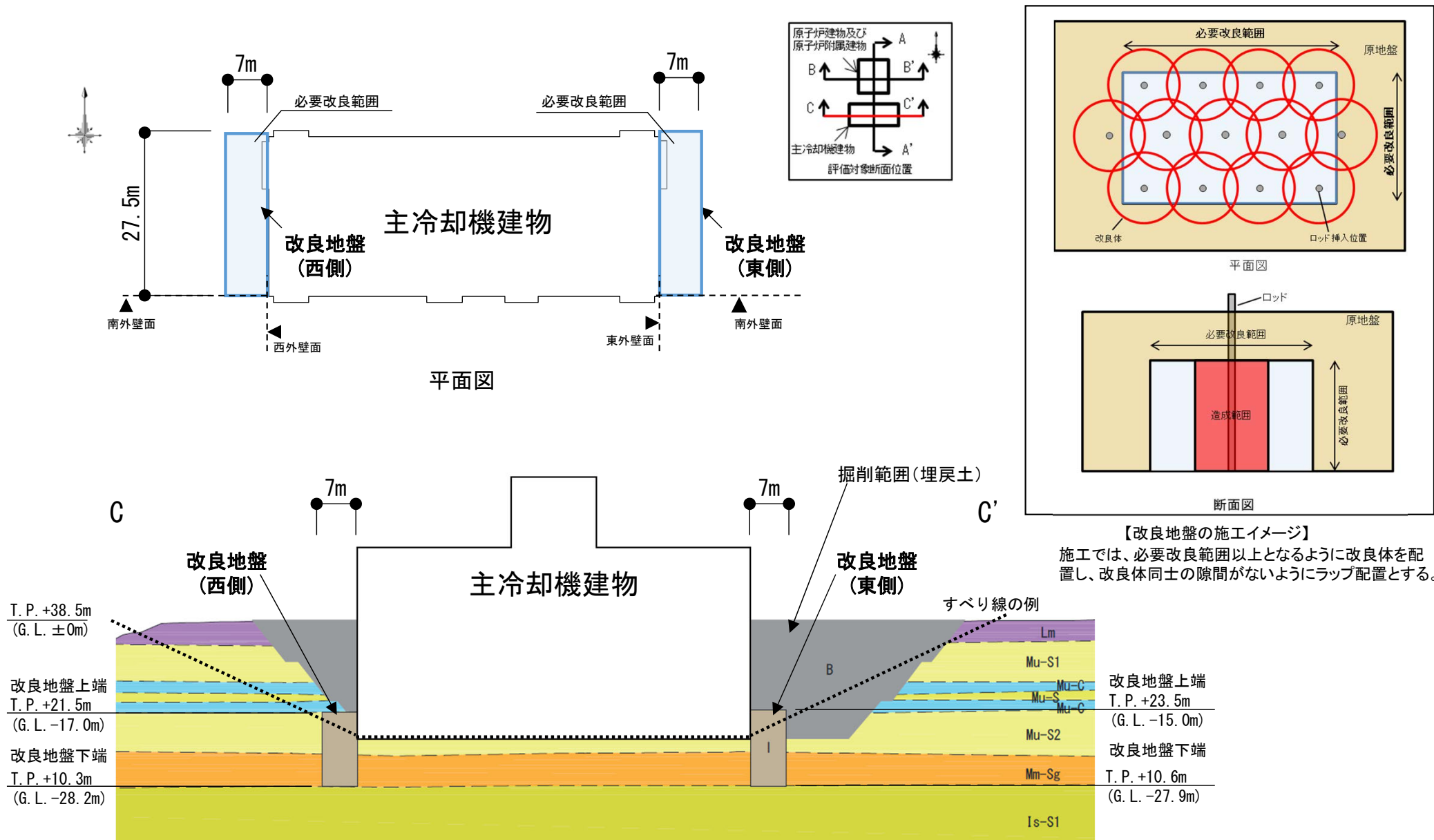
図 断面図 (東西 C-C' 断面)
