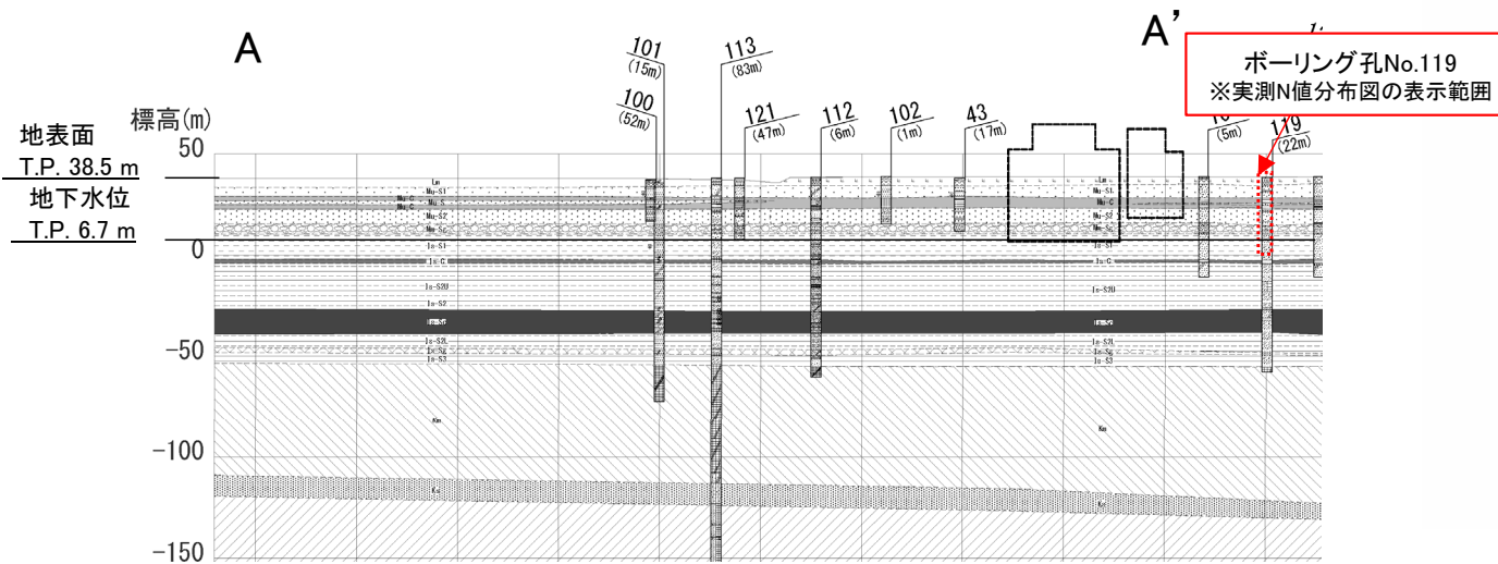
地質断面図(A-A'断面)
