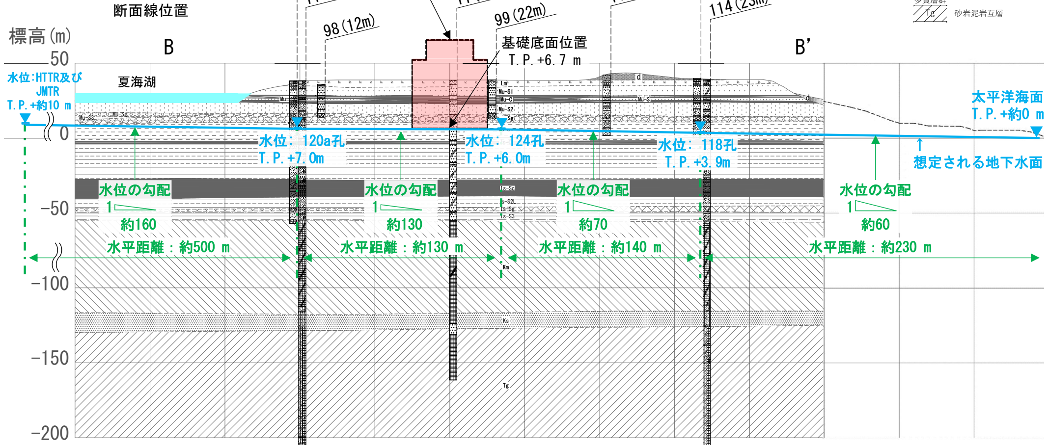
B-B'断面(東西方向)
