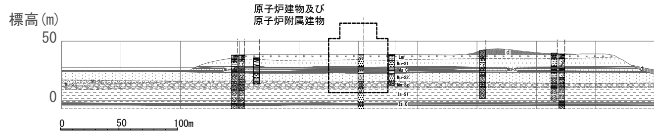
B-B' 断面図
