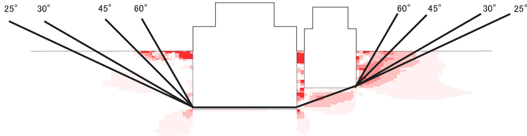
せん断応力比分布
