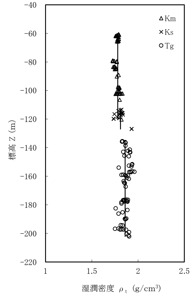
湿潤密度試験結果 (Km、Ks、Tg)
