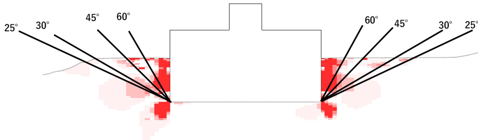
せん断応力比分布
