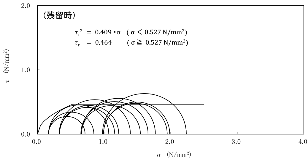
強度特性(Is-C)
