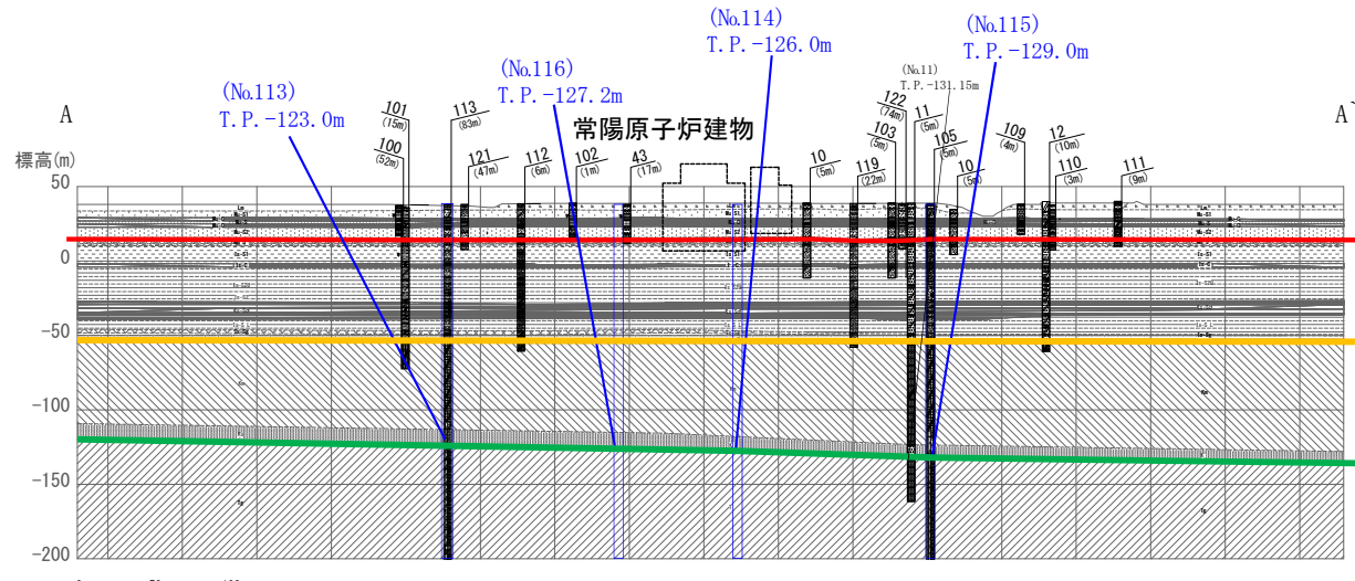
A-A' 測線（南北方向）
