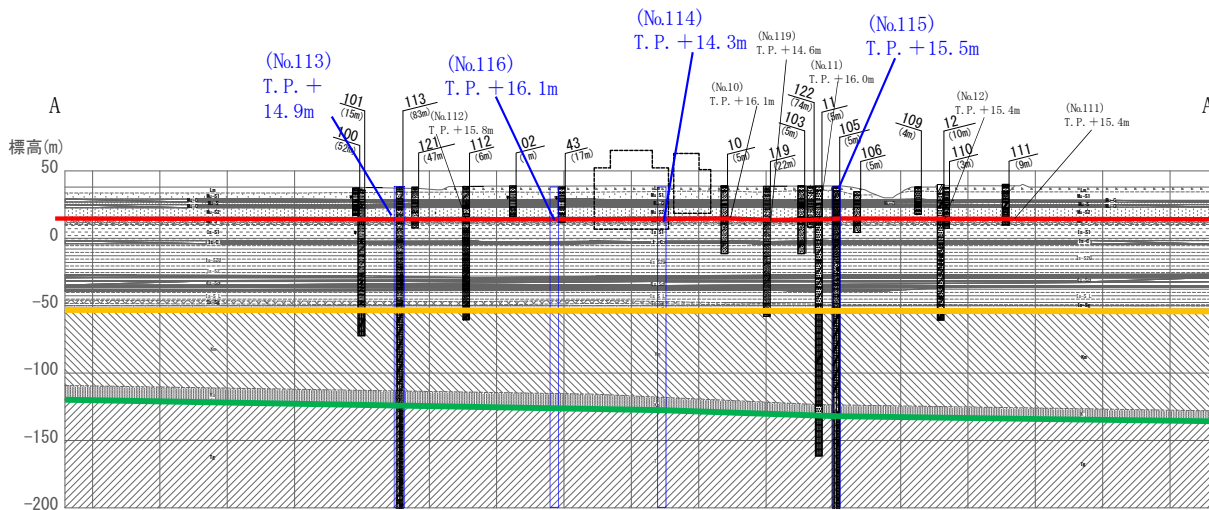
A-A' 測線 (南北方向)
