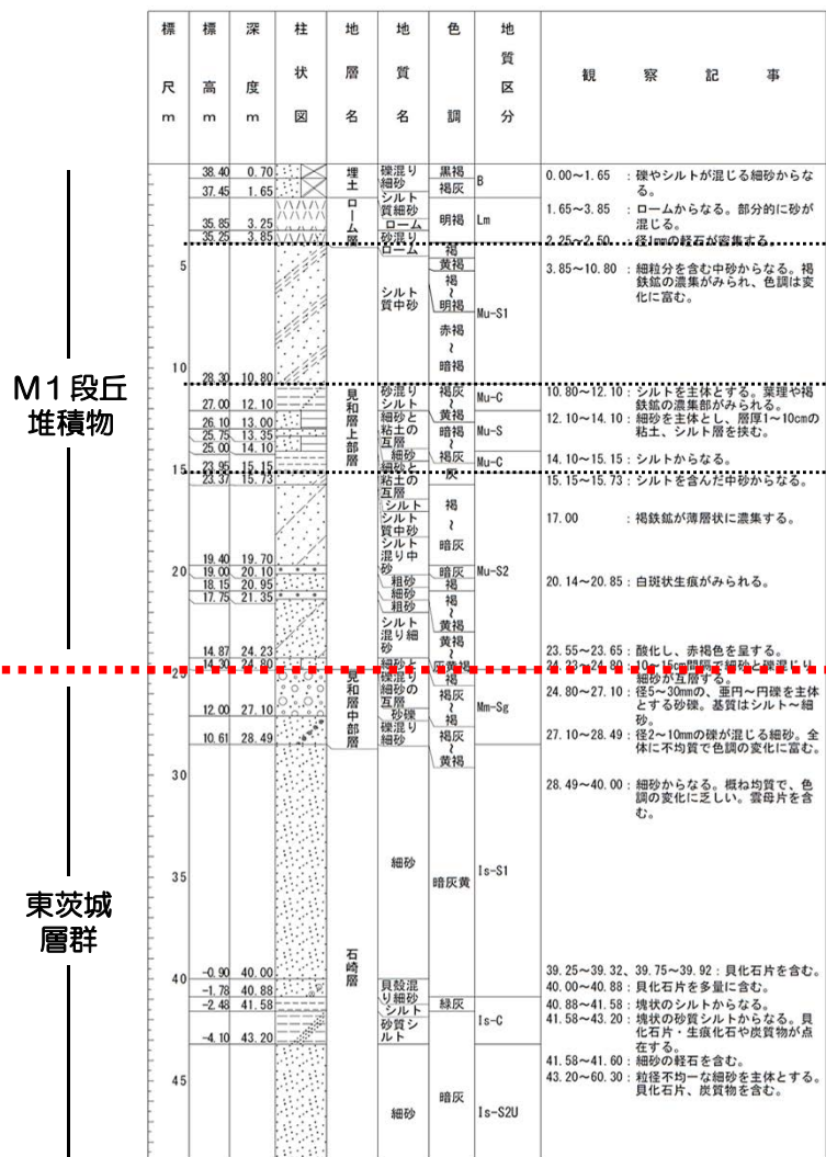
敷地内ボーリング柱状図 (No.114)
