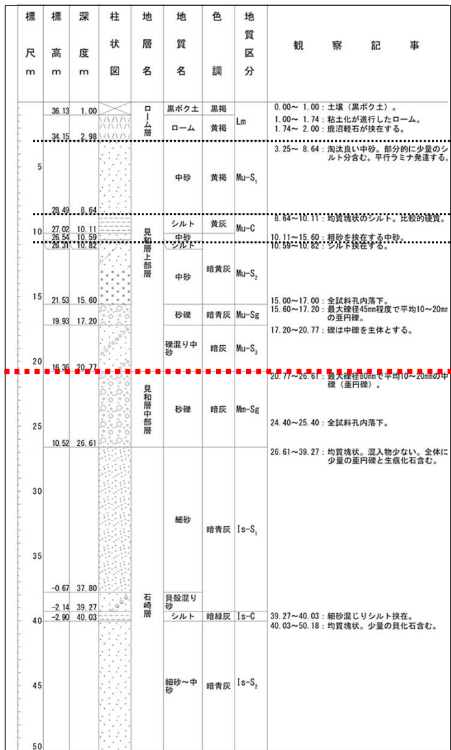
敷地内ボーリング柱状図（No.3）
