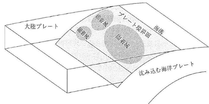
図 プレート境界面の固着状態を示す模式図 (出典：「津波の辞典」，首藤他，朝倉書店，2007)
