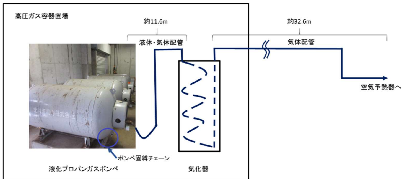
図 雑固体焼却炉のプロパンガス概略系統図
