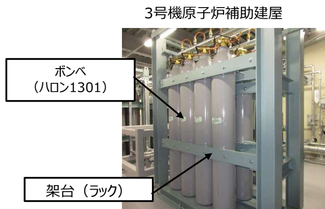
図 発電所におけるボンベの設置状況
