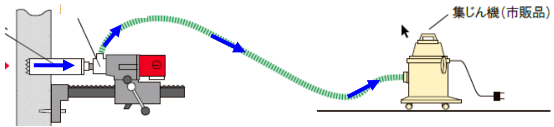
コア抜きドリルから集塵機の構成図
