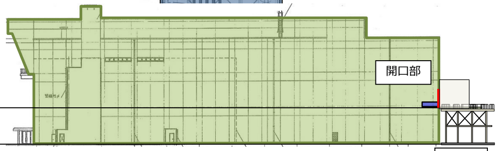
図：7号主建屋（西側立面図）
