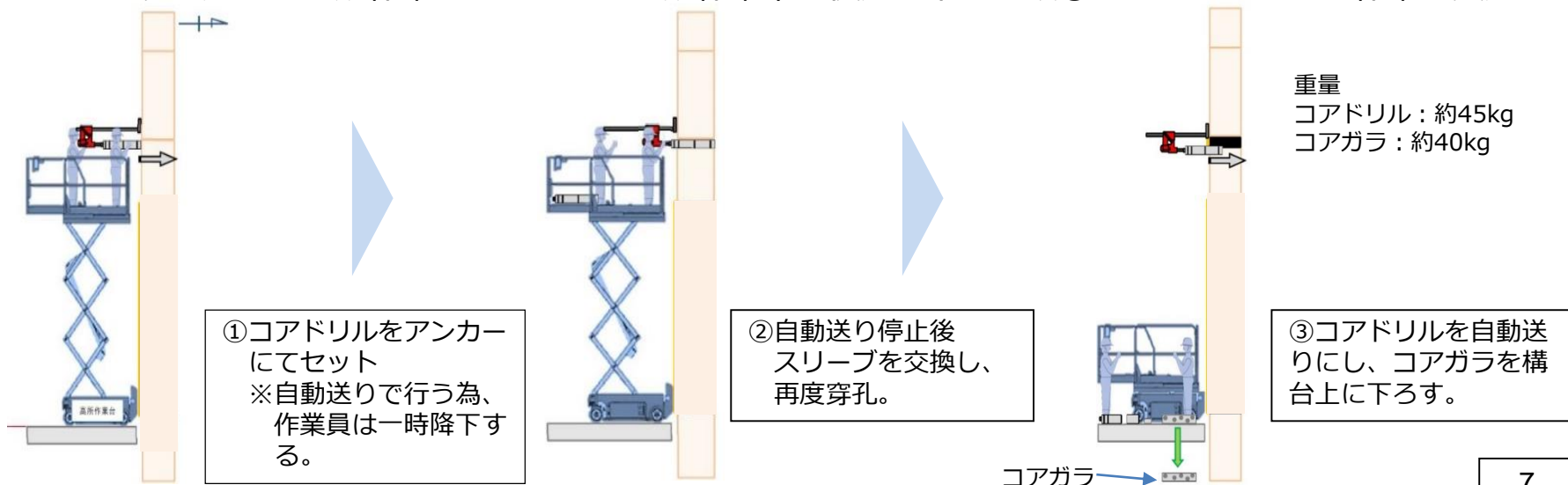
コアドリル
