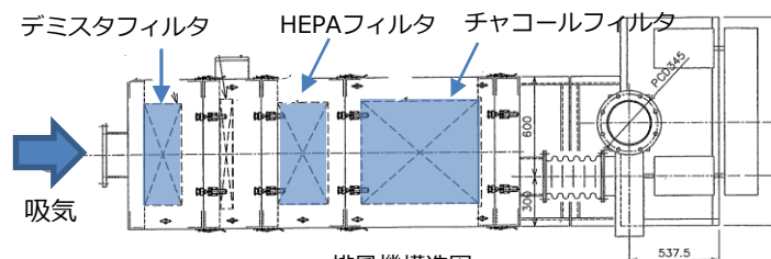
排風機構造図
