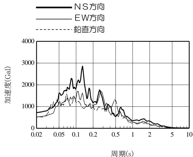
(加速度応答スペクトル, h=5%)
