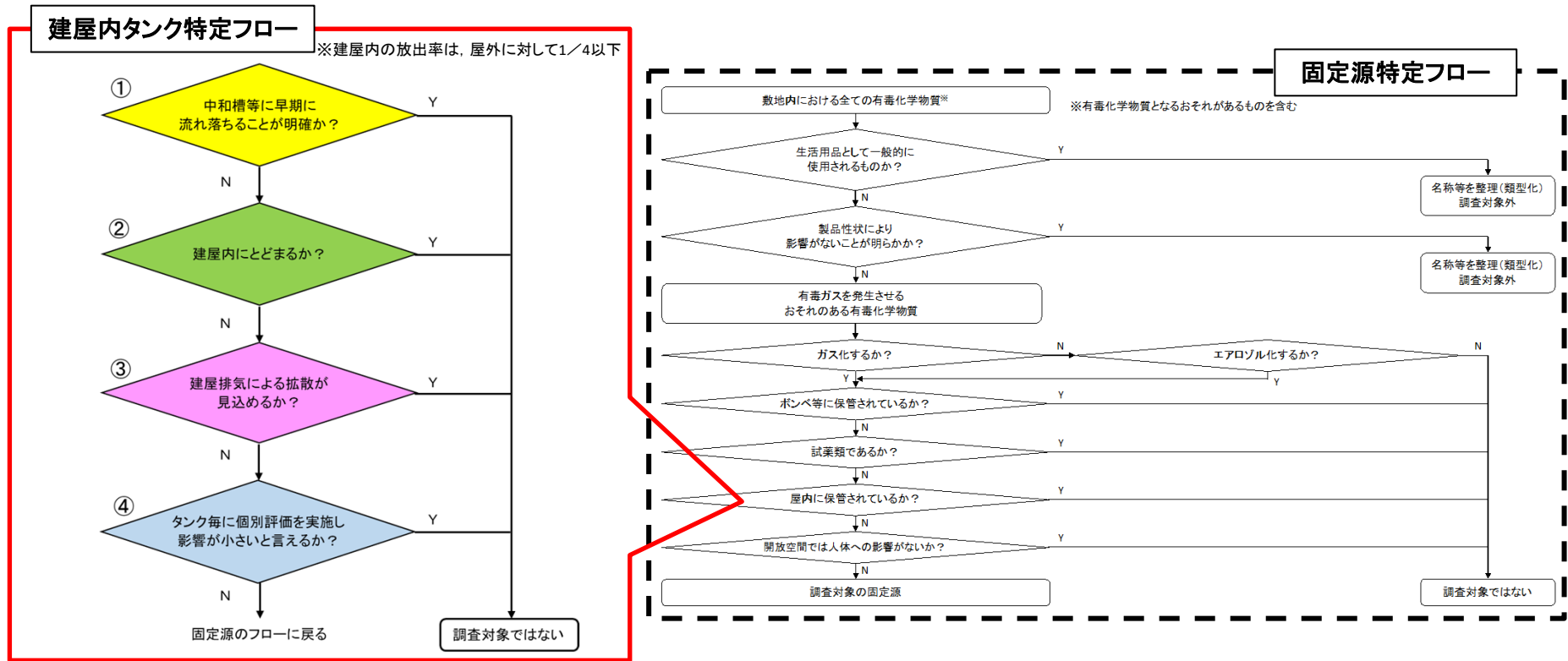
図23 建屋内タンク特定フロー
