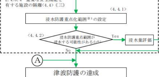
図1 津波による損傷防止の確認フロー
