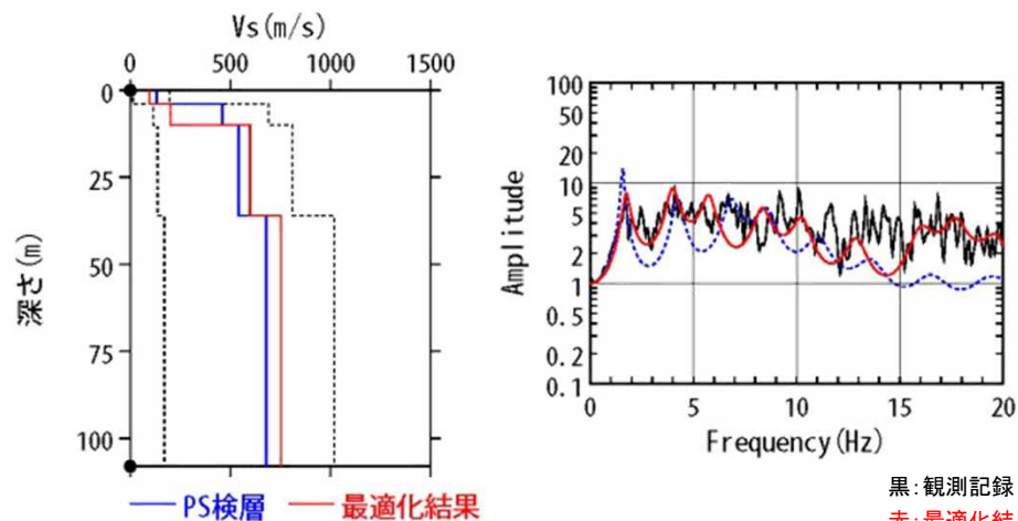
伝達関数の比較(水平)
