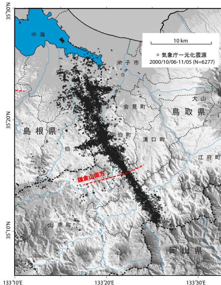
震央分布図
