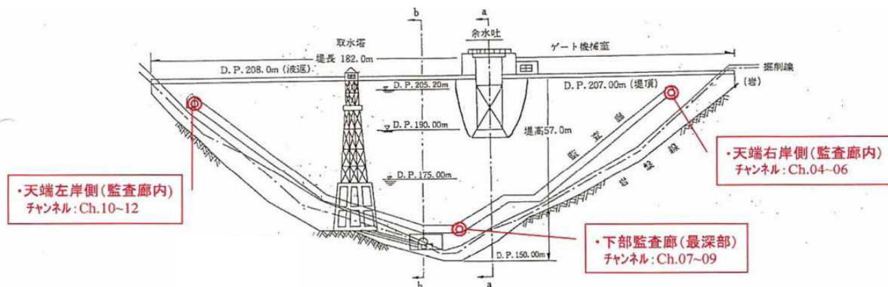
地震観測位置(断面図)
