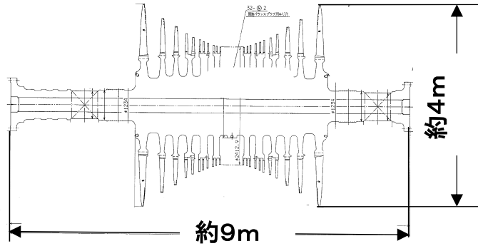
2号 低圧タービンローター 85.3t
