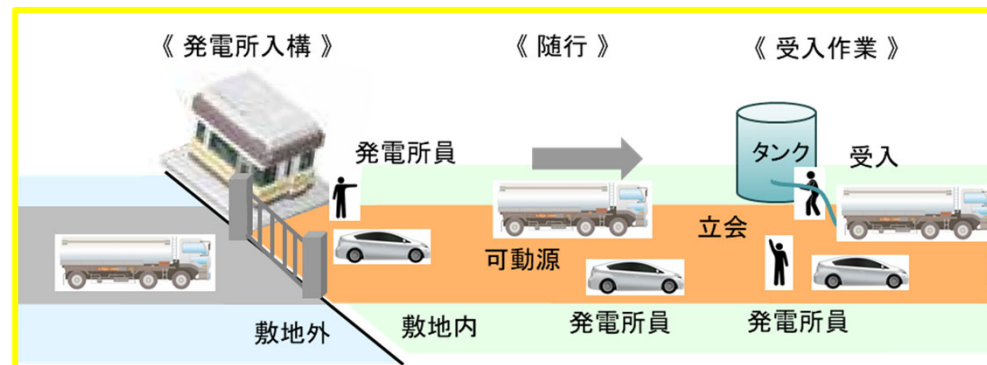
図11 有毒ガスの発生の検出のための実施体制
