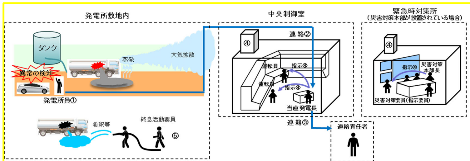
図12 漏えい時の防護措置の流れ
