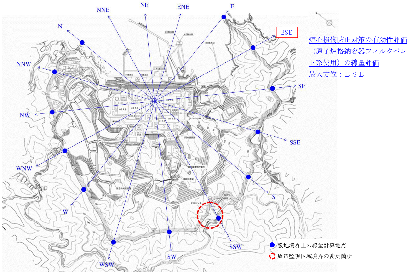
図 2-4(1) 炉心損傷防止対策の有効性評価 (原子炉格納容器フィルタベント系使用) の線量計算地点及び実効線量 (最大値) の方位
