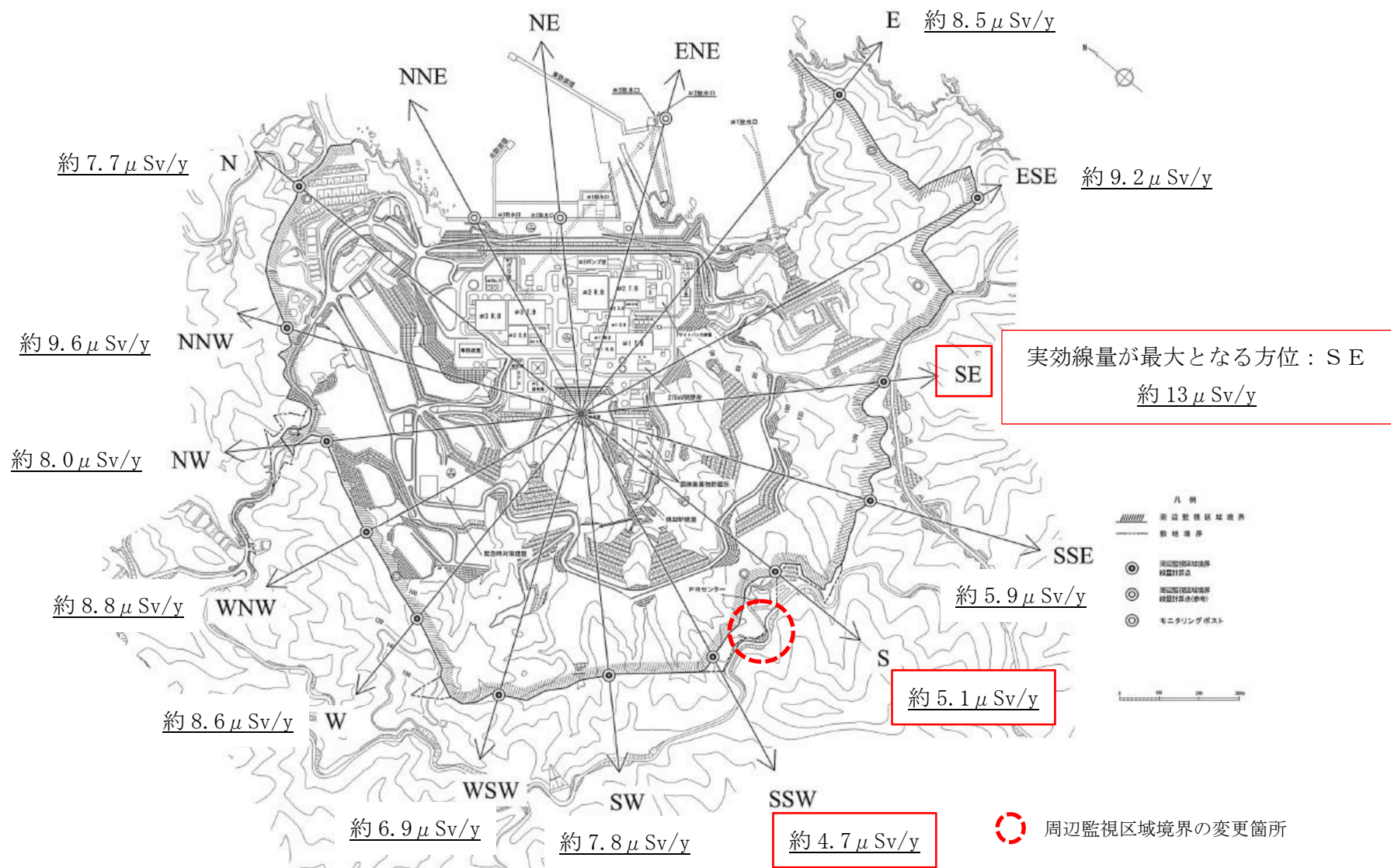
図 2-2(1) 気体廃棄物の希ガスのγ線による実効線量（陸側 13 方位）
