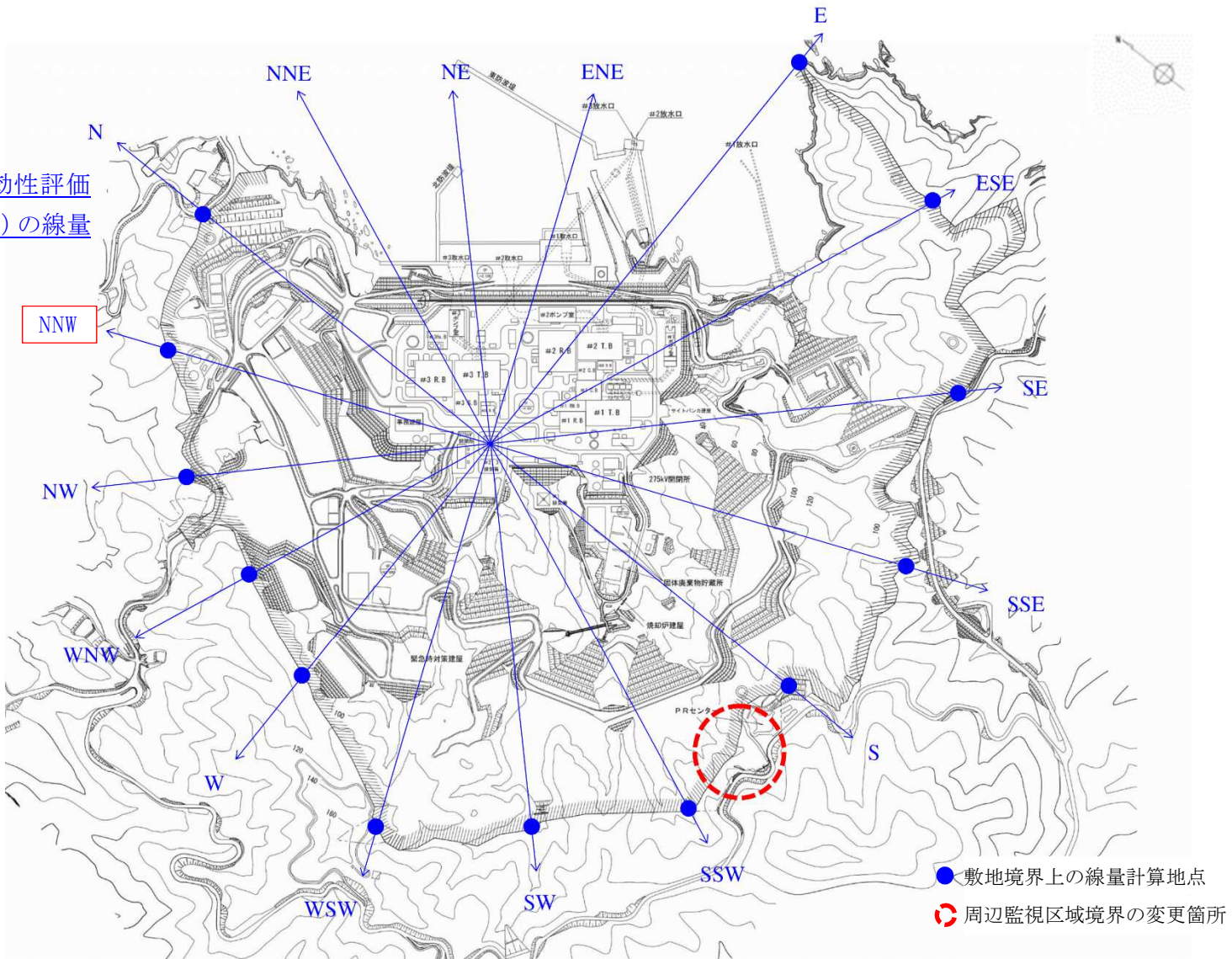
図 2-4(2) 炉心損傷防止対策の有効性評価 (耐圧強化ベント系使用) の線量計算地点及び実効線量 (最大値) の方位
