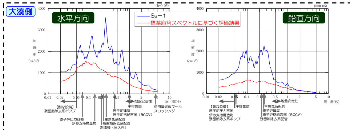
第39-4-1図 既設機器の固有周期（第9回標準応答スペクトルの規制への取り入れに伴う設置許可申請等の要否に係る会合(2022年2月18日)資料1より抜粋)
