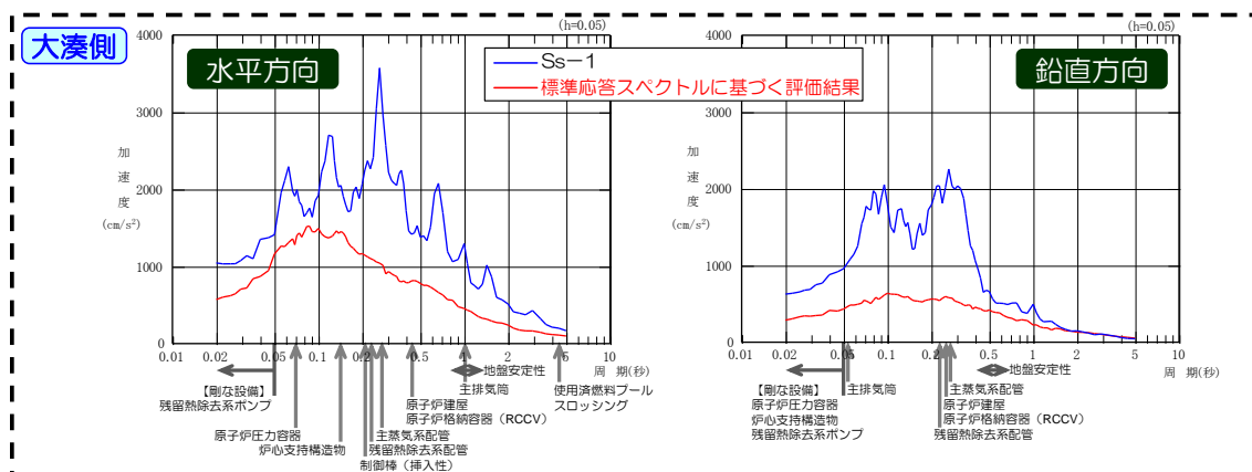
第39-4-1図 既設機器の固有周期（第9回標準応答スペクトルの規制への取り入れに伴う設置許可申請等の要否に係る会合(2022年2月18日)資料1より抜粋)
