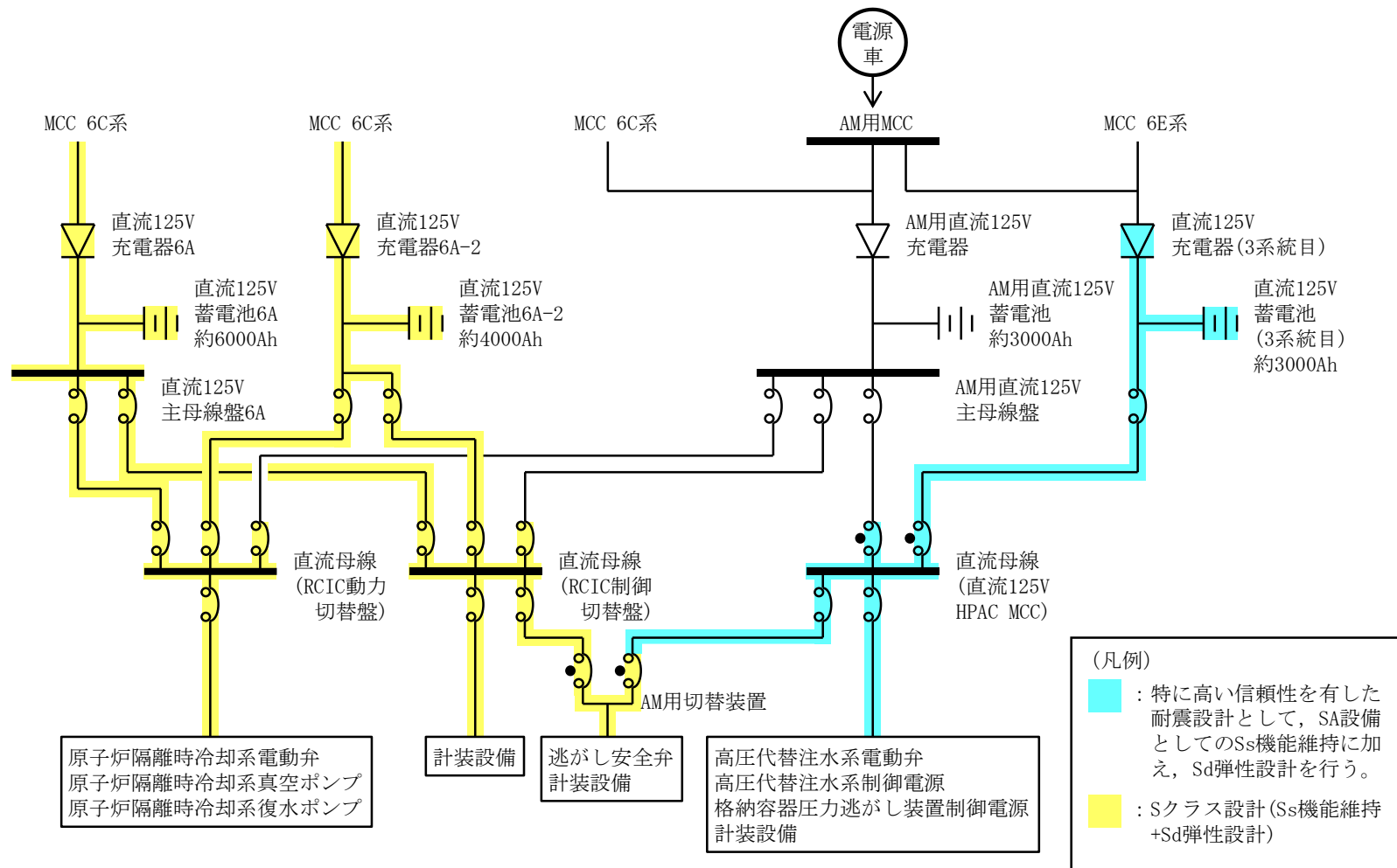
第 57-4-5 図 特に高い信頼性を有した電源設備の耐震設計範囲 (6号炉)
