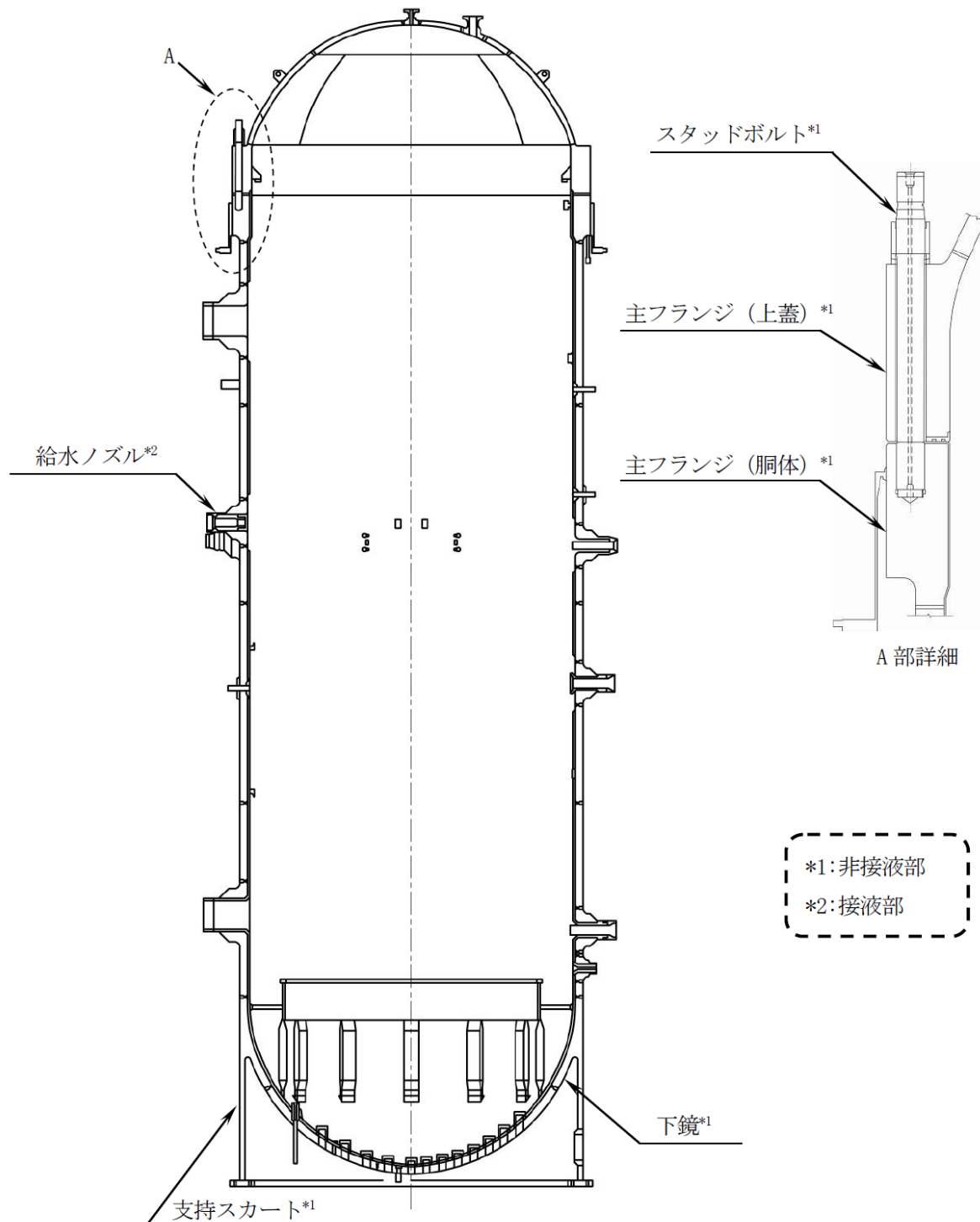
図2 原子炉圧力容器の評価対象部位
