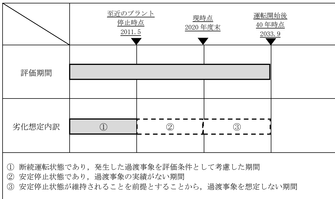
図 1-1 安定停止の維持状態での劣化想定の内訳
