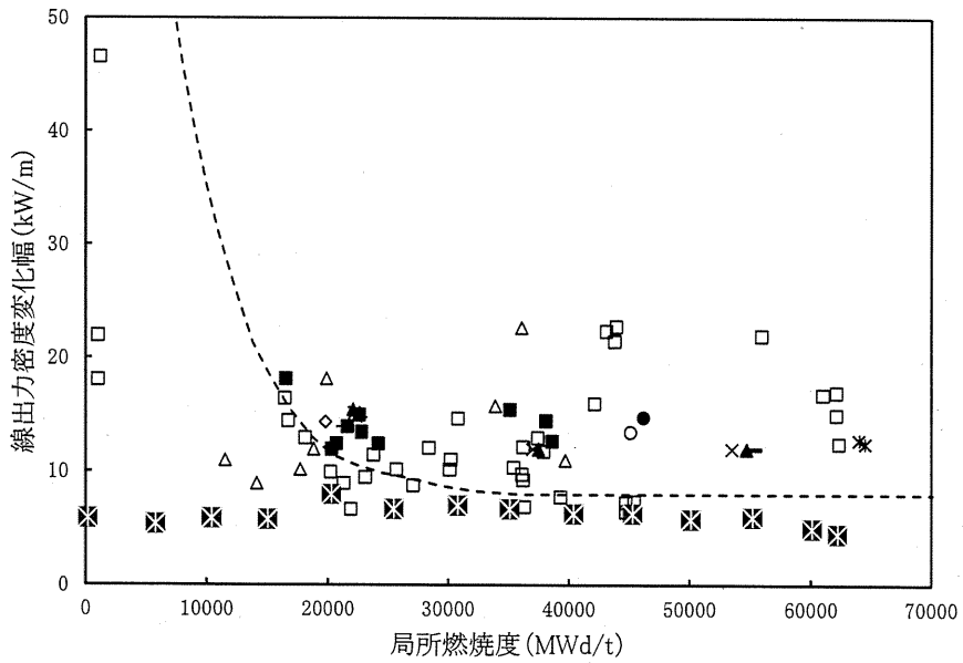
第3-16図 (1) 被覆管の出力ランプ試験結果 (最大線出力密度が最大の場合の出力変化)
