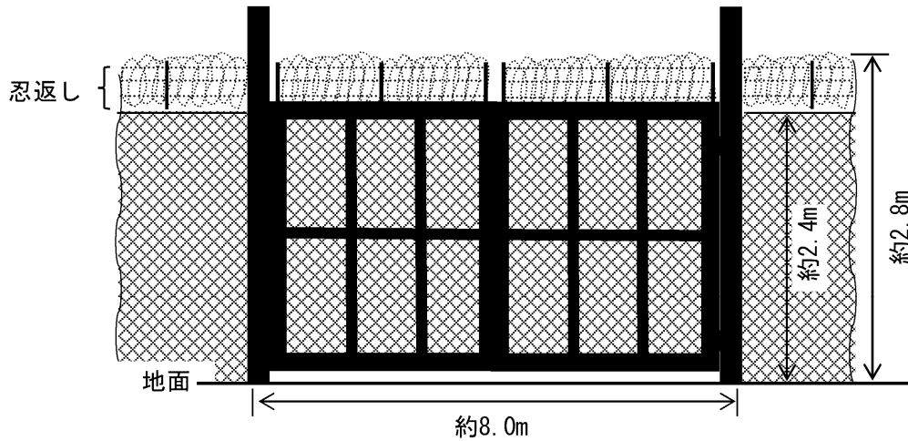
図2 新設する門扉の設置正面図
