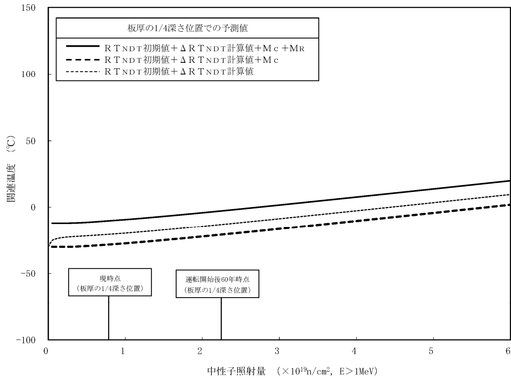
図4 原子炉容器胴部（炉心領域部）の中性子照射脆化に対する 関連温度の国内脆化予測法による予測と監視試験結果の関係
