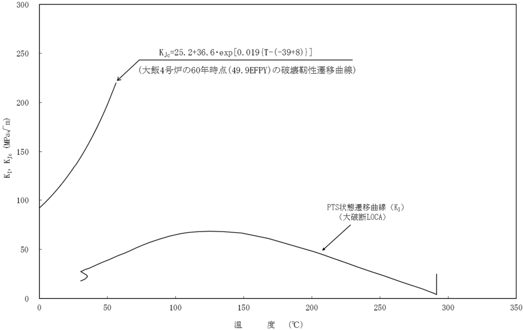
図参考 1-1 JEAC4206-2016 を用いた PTS 評価結果
