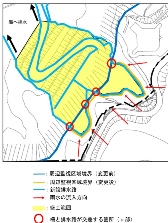
図3 周辺監視区域柵と排水路配置の関係
