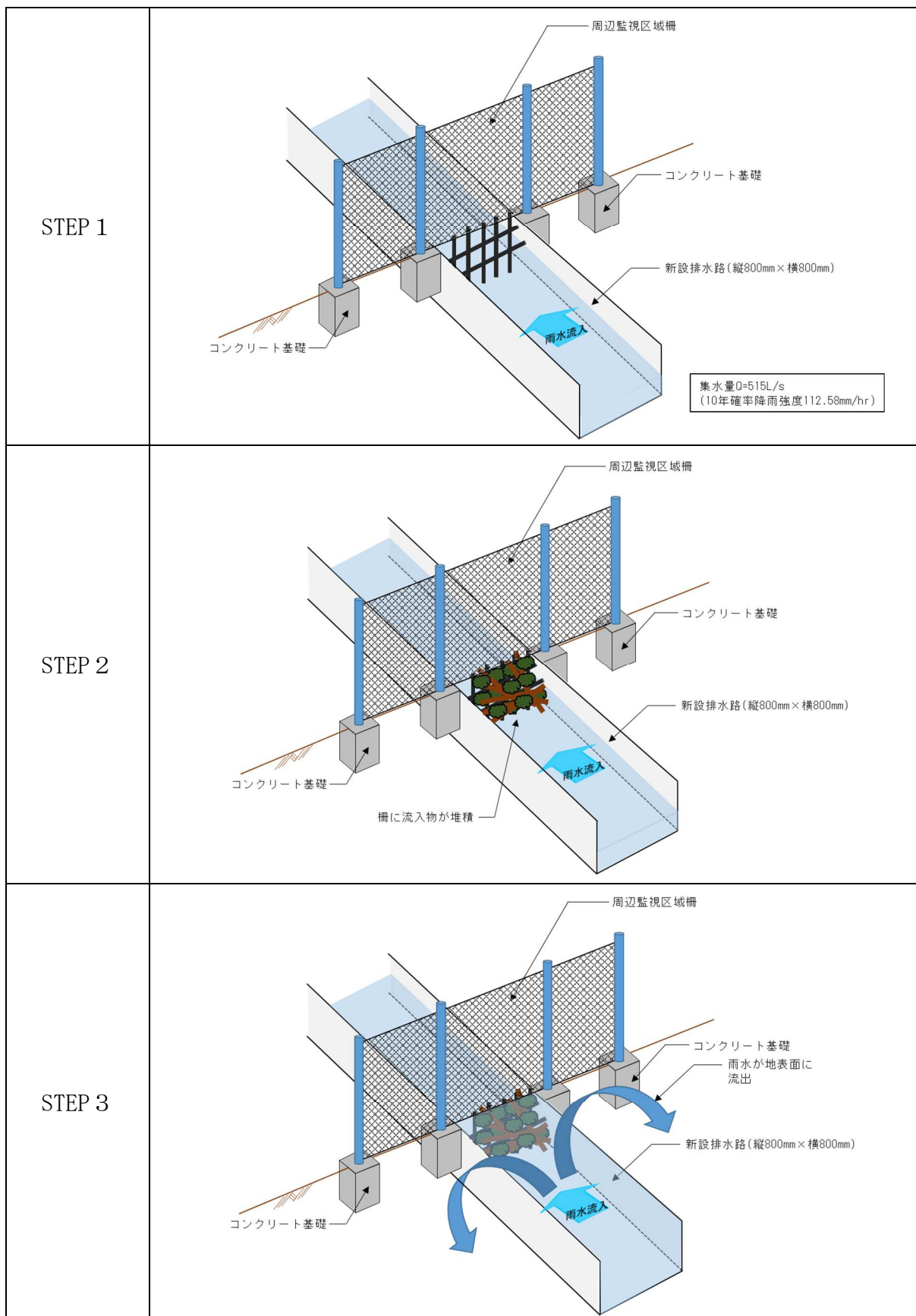
図4 溢水が想定される箇所（a部）の状況イメージ
