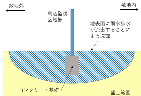
図6 洗掘概要A—A断面
