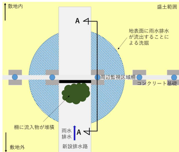
図5 洗掘概要平面
