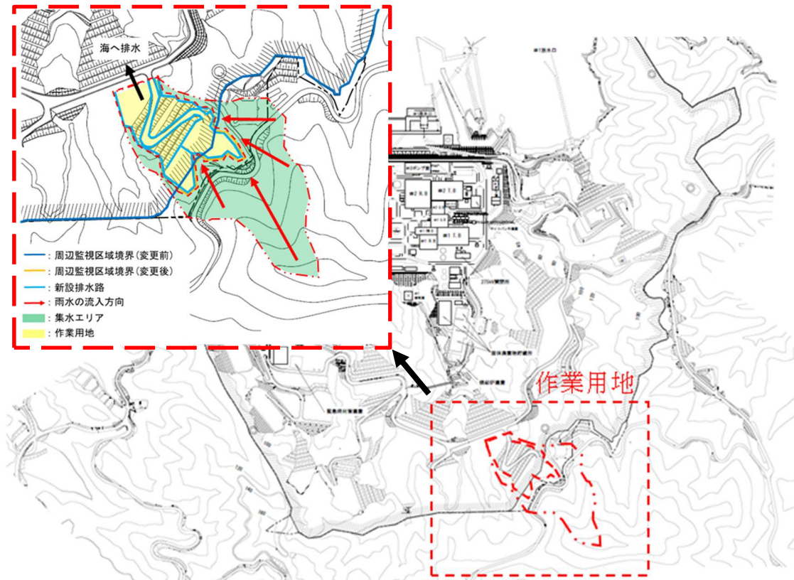
図1 周辺監視区域柵および排水路計画平面
