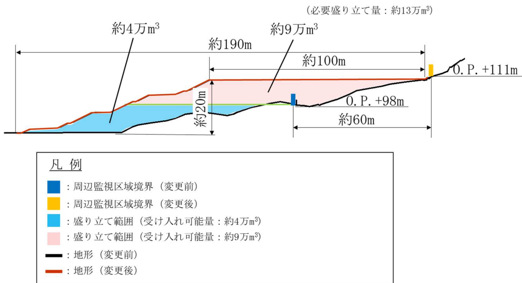
図5 作業用地拡大箇所の縦断図 (A-A 矢視)
