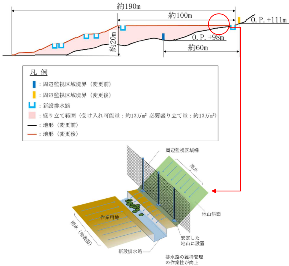
図2 周辺監視区域柵および排水路計画断面図・鳥瞰図
