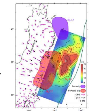
長期的なスロースリップの発生領域 (Yokota and Koketsu (2015))
