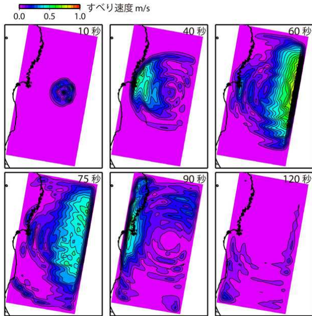
(左図)コンター:総すべり量の分布, 0309:前震(Mw7.3)のメカニズム, MS:本震のメカニズム, 0312及び0314:余震(それぞれMw6.5,Mw6.1)のメカニズム, 青点:前震の震央, 赤点:余震の震央, グラフ:地震モーメントの放出速度の推移 (右図)すべり速度分布のスナップショット
