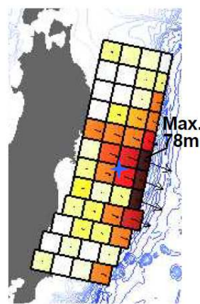
すべり量分布(合計)
