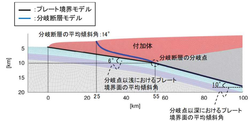
【南海トラフ沿いにおける分岐断層の地殻変動量分布】
