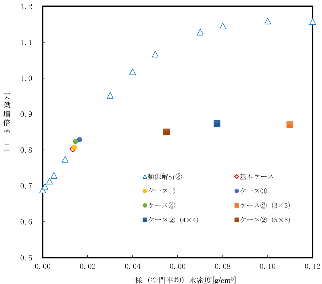
第3-3図 基本ケース、感度解析ケース（水位0cm）および類似解析③の実効増倍率（ケース②での空間平均水密度は、局所範囲内において一様水密度に換算した値）
