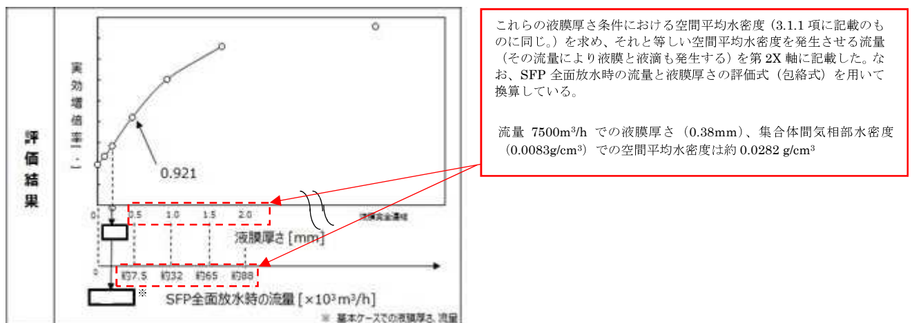
図2 燃料集合体の中のみを変化させるパラメータスタディ 評価結果
