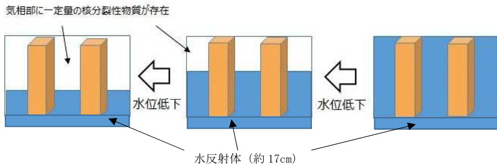
第 3-4-2 図 TCA 実験炉の体系概念図（燃料領域＋下部反射体）
