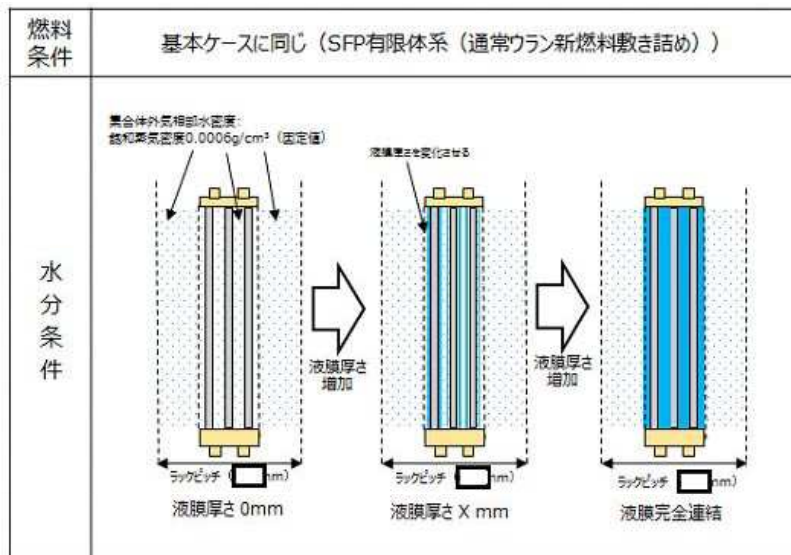
図1 燃料集合体の中の水密度のみを変化させるパラメータスタディ 評価条件
