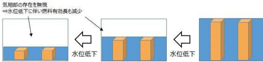
第 3-4-1 図 ①、②式に基づく評価で考慮する体系の概念図（下部反射体は無い）
