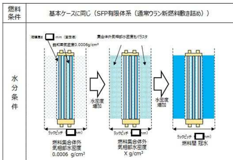
図3 燃料集合体の外の水密度のみを変化させるパラメータスタディ 評価条件
