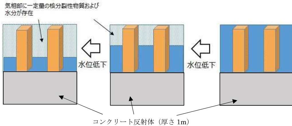
第 3-4-3 図 基本ケースの体系概念図（燃料領域＋下部反射体）
