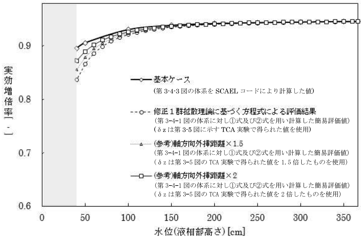
第3-6図 修正1群拡散理論に基づく方程式より求まる実効増倍率
