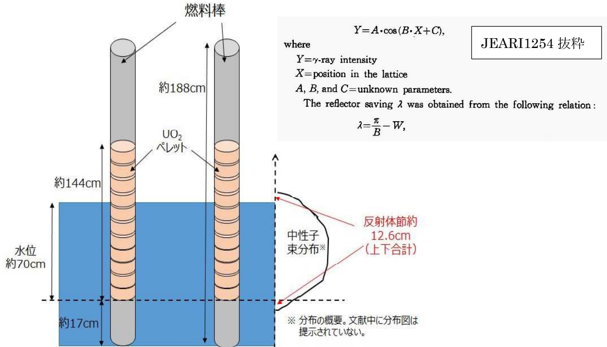
第3-5図 文献（JEARI 1254）に示される軸方向外挿距離取得時の測定体系
