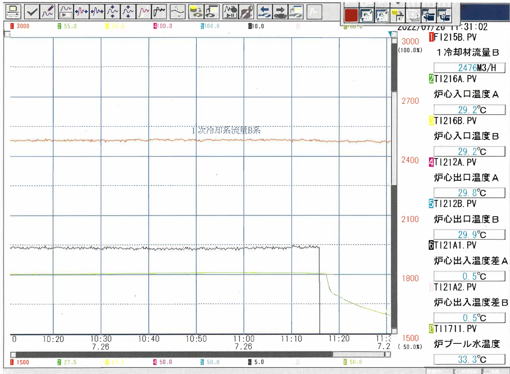
1次冷却系流量B系のトレンドデータ
