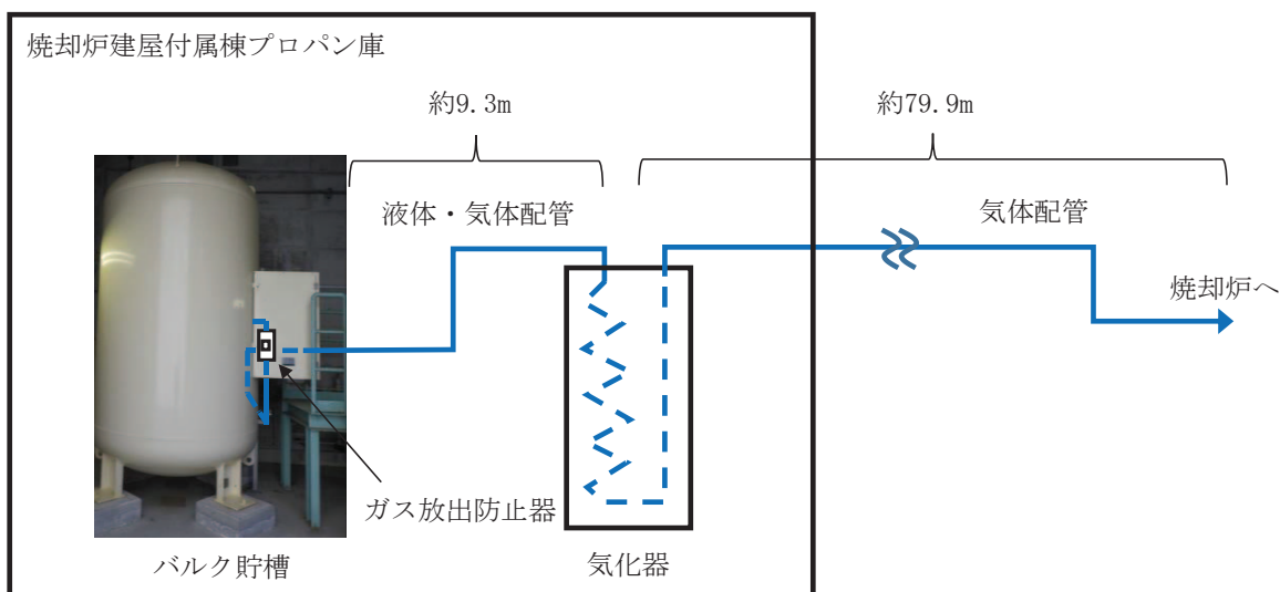
図1 廃棄物焼却設備のプロパンガス概略系統図
